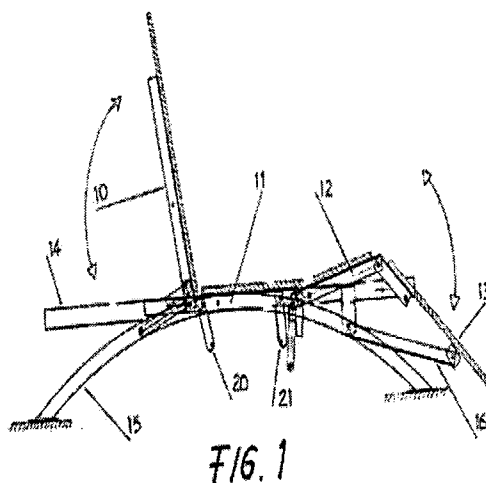
Figura de la solicitud de patente de invención denominada "cama eléctrica ajustable con soporte en arco convertible en silla" solicitada el 26 de enero de 2007.
