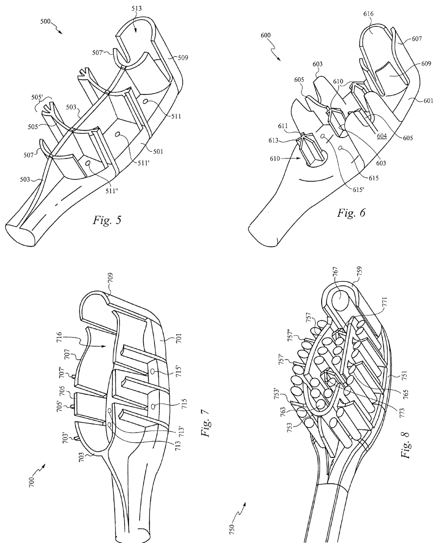
Figs. 5, 6, 7 y 8 del documento US 6,859,969
