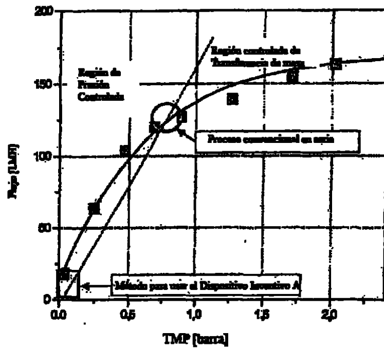
Figura 9: Ejemplo de curva de presión-flujo (flujo de permeato específico en LMF = litros/hora/m 2 sobre presión de transmembrana) y determinación del punto de funcionamiento. El círculo muestra el punto de funcionamiento típico que se ajustará mediante TMP para procesos en serie convencionales. El rectángulo muestra la región operacional que se ajustará mediante bomba de permeato según el método para utilizar el dispositivo inventivo A.
