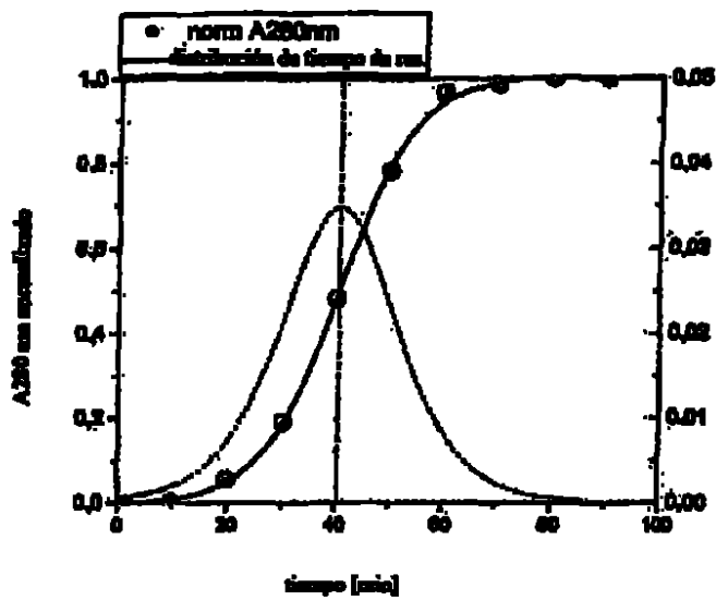
Figura 10: Ejemplo de distribución de tiempo de residencia y tiempo de residencia medio del sistema continuo integrado UF (300) como método para utilizar el dispositivo inactivo. Método para el sistema continuo descrito con caudal de 290 cm 3 (62,5 cm de longitud), 130 LMH de flujo cruzado, 02 LMH de flujo de retención, 2 LMH de flujo de permeato.
