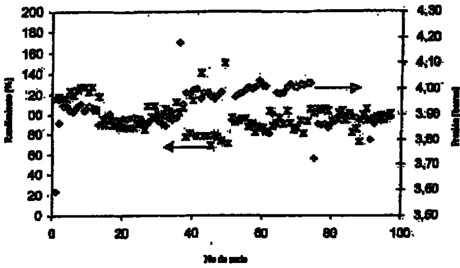
Figura 15: Ejemplo de resultados a largo plazo del dispositivo inventivo B. Rendimiento y disminución de pérdida cercana a 100 ciclos de aducción/desucción consecutivas con el aductor/conector (prototipo objetivo: versión de factor 2/UMI) (comparación de configuración presentada por la patente global; aductor/conector: aductor comercial, Manning Q, Roll Corporation).
