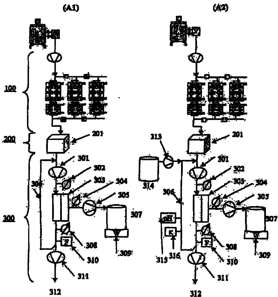
Figura 1 Representación esquemática de 2 incorporaciones de un dispositivo inventivo A para fabricación continua, integrada y estática. Representación esquemática A1 mostrada en el lateral izquierdo y representación esquemática de la incorporación A2 mostrada en el lateral derecho.
