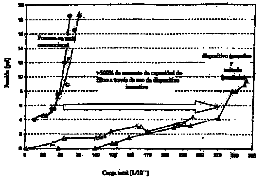
Figura 8: Comparación ejemplar de las capacidades de carga total por 10'' de espesor de filtro para proceso convencional en serie e incorporación del dispositivo inventivo y método para la extracción de partícula continua (proceso de filtración continua integrada) utilizando cápsulas de filtro comercial idénticas. Método ejemplar que produce Factor VIII recombinante de capacidad mostrada.
