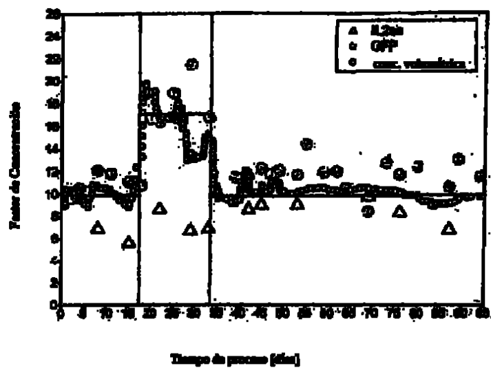
Figura 14: Ejemplo de resultados a largo plazo del dispositivo inventivo A directamente acoplado a fluorescencia por perfusión de productos proteicos de expresión celular 2 (GFP de proteína fluorescente verde y IL-2SA). 10 MD de membranas se ha utilizado. El factor de concentración de los productos proteicos, según determinado por los ensayos específicos, y el factor de concentración viral total se muestra como función de tiempo de proceso continuo.
