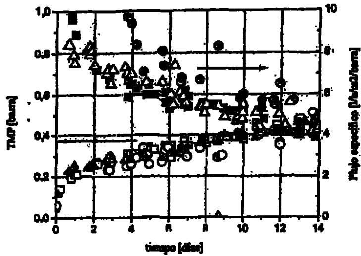
Figura 1.2: Ejemplos de rendimiento del dispositivo inventivo A. Presión de transmembrana y flujo específico del sistema de ultrafiltración integrado continuo (300) como una función del tiempo de proceso continuo para 3 ejemplos diferentes mostrados. Triángulos = 100 kD de membrana, Factor VIII (rFVIII) monómero de coagulación; Cuadrados = 10 kD de membrana, interferencia-2 recombinante; Círculos = 50 kD de membrana, glicoproteína generada por ingeniería genética ( M_r > 100 kD). Todos los ejemplos mostrados son alimentación por perfusión continua libre de plasma-proteína.
