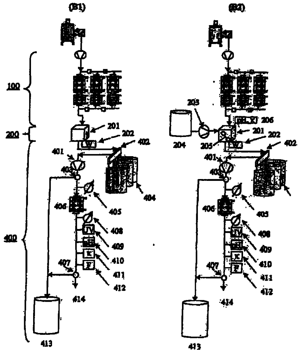
Figura 3: Representación esquemática de 2 incorporaciones de un dispositivo inventivo B para fabricación continua, integrada y en serie. Representación esquemática B1 mostrada en el lateral izquierdo y representación esquemática de la incorporación B2 mostrada en el lateral derecho.
