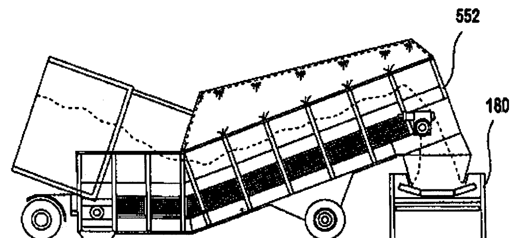
FIG. 2B (TECNICA PREVIA)
