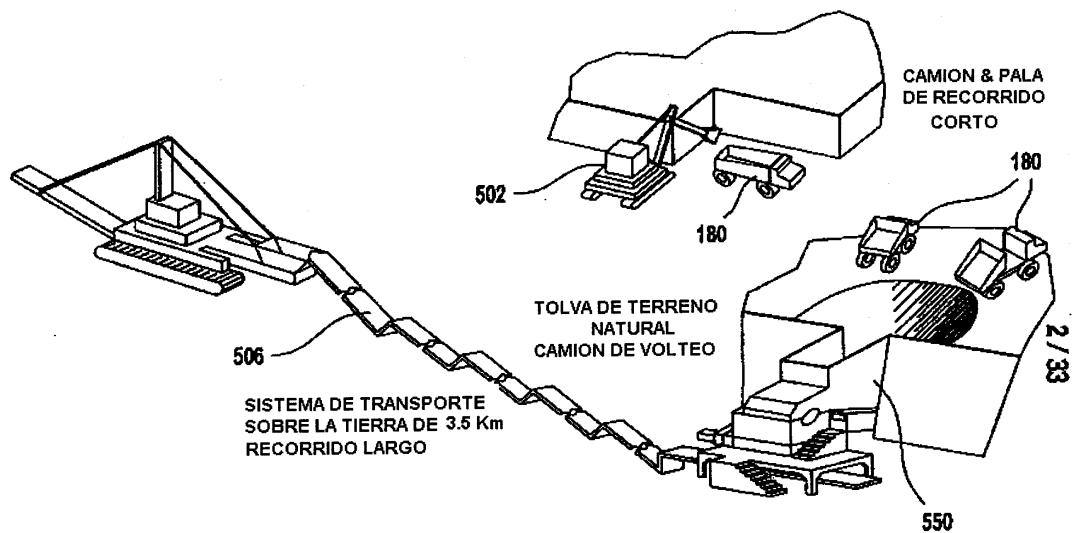
FIG. 1 B (TECNICA PREVIA)
