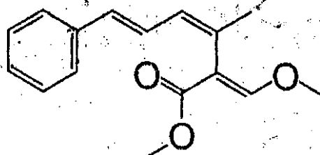
Strobilurin A
