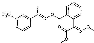
trifloxystrobin CGA 279202
