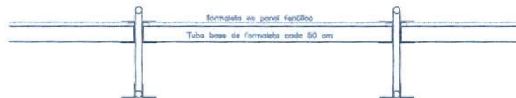
SECCION TRANSVERSAL ARMAZO JOIST PREVIO A FUNDIDA
