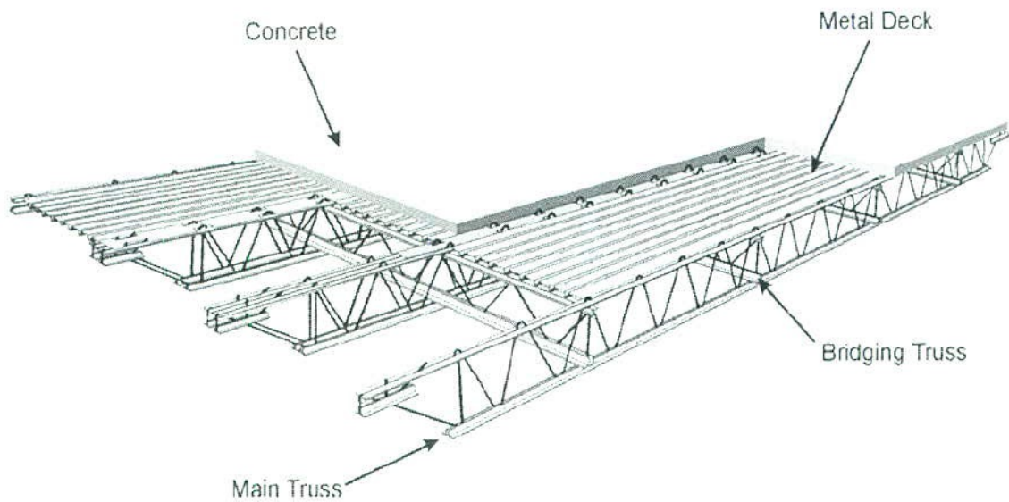
Figura N°1: Joist con conectores de Cortante que forman parte de la Celosía
