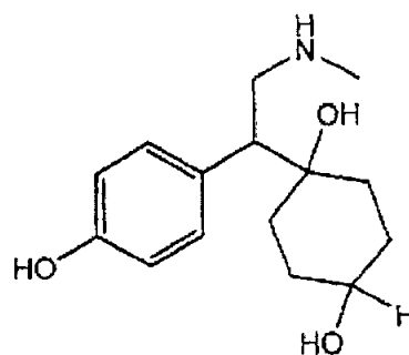
N-Demetilación PM=265, RRT=0.98
