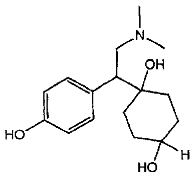
1-[2-dimetilamino-1-(4-fenol)etil] -cis-1,4-ciclohexandiol PM=279, RRT=1.00
