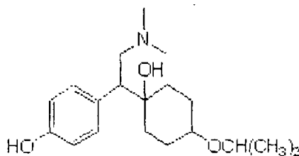
4-[2-Dimetilamino-1-(1-hidroxi-4-isopropoxi-ciclohexil)-etil]-fenol
