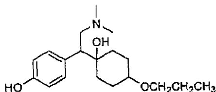
4-[2-Dimetilamino-1-(1-hidroxi-4-propoxi-ciclohexil)-etil]-fenol
