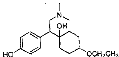
4-[2-Dimetilamino-1-(4-etoxi-1-hidroxi-1-ciclohexil)-etil]-fenol
