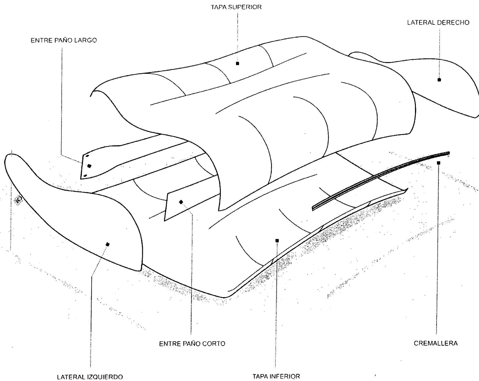
GRÁFICO 3. Explosión General
