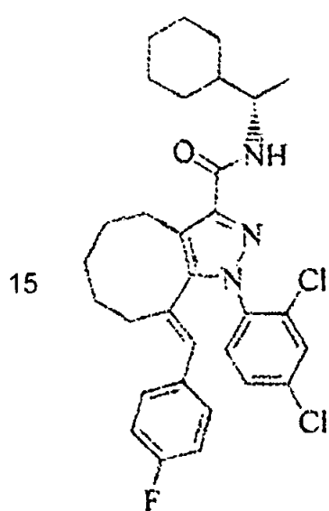
Compuesto 16
