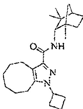
Compuesto 8
