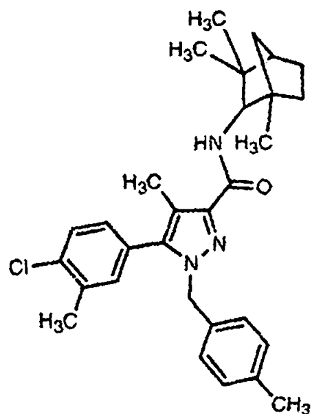
SR 144528
