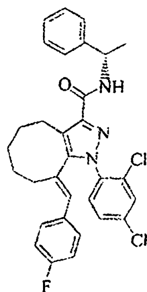
Compuesto 15
