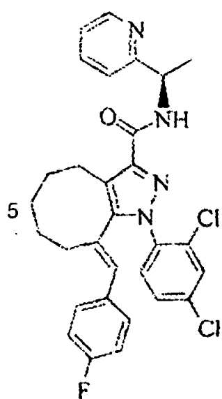
Compuesto 13
