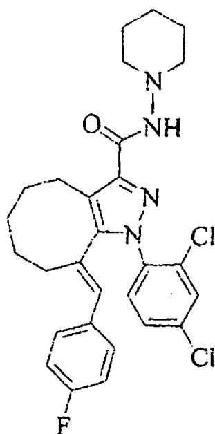
Compuesto 19
