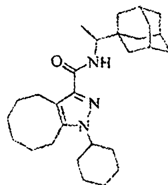
Compuesto 6
