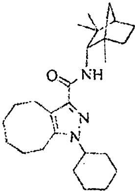
Compuesto 1
