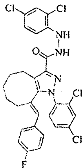
Compuesto 11
