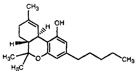
THC
