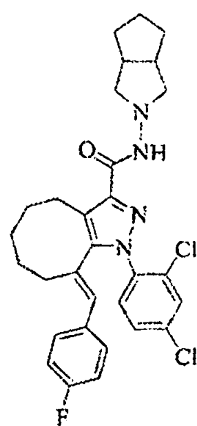
Compuesto 18
