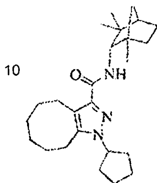
Compuesto 7
