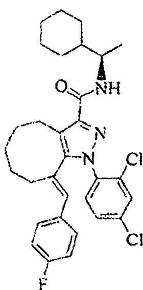
Compuesto 17
