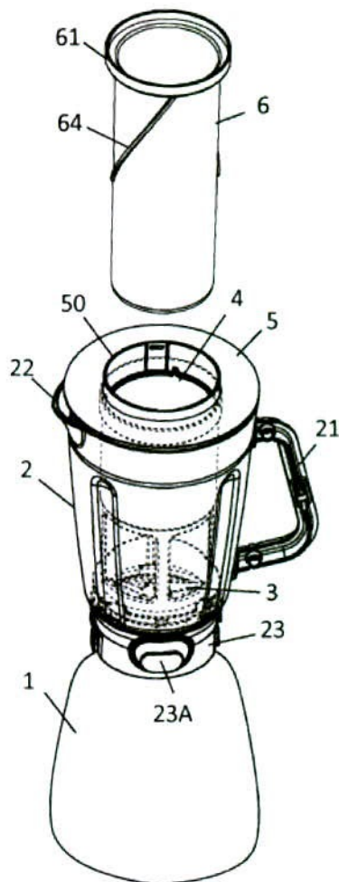
Vista en perspectiva de un aparato de preparación culinaria conforme a un modo particular de realización de la materia mencionada en la solicitud de patente colombiana CO 14-070.346
