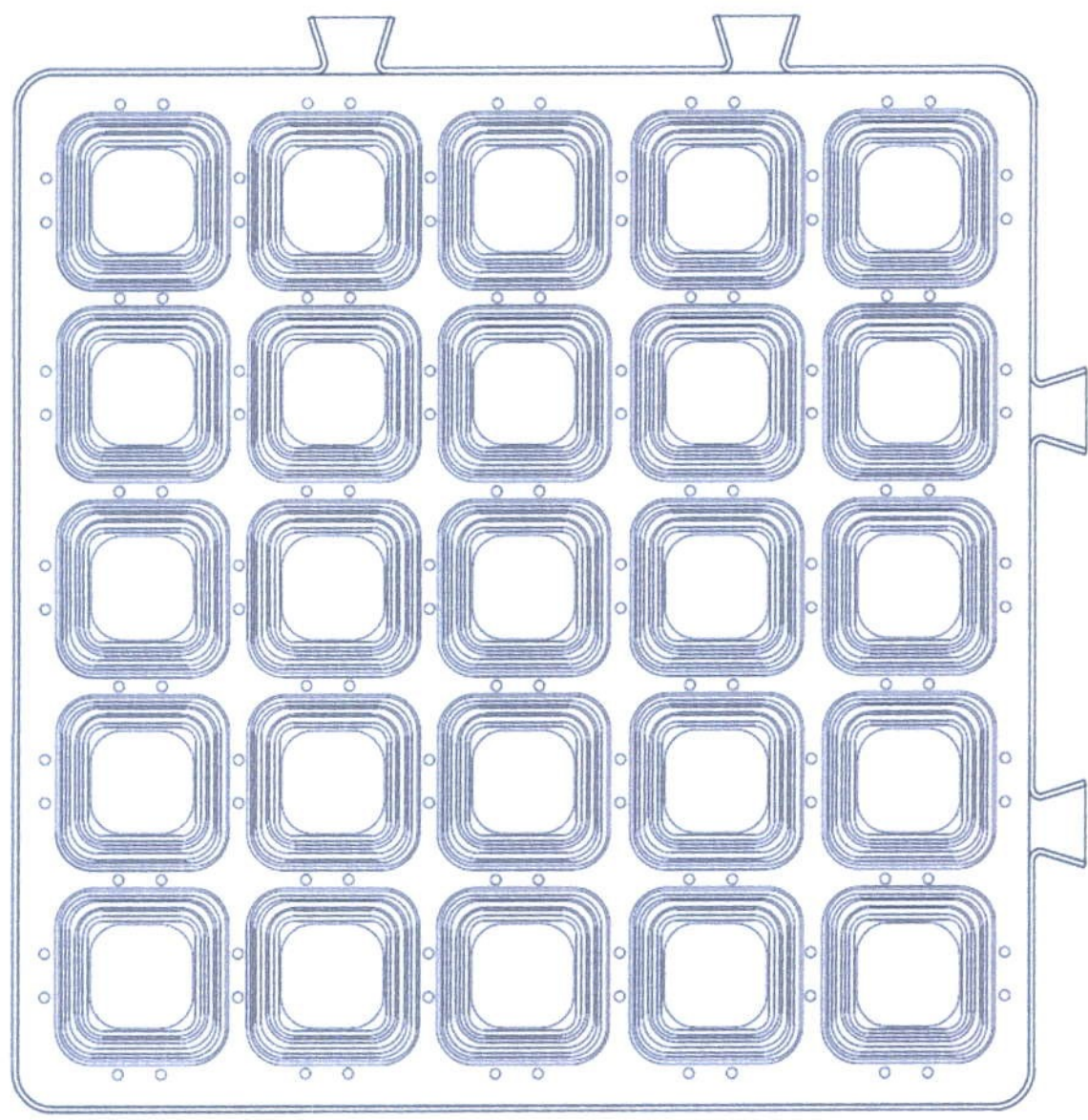
Figura 4: Muestra planimetría vista en planta de la Bandeja almacenadora de agua para cubiertas y terrazas vegetales y/o verdes.
