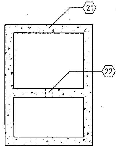
CORTE
