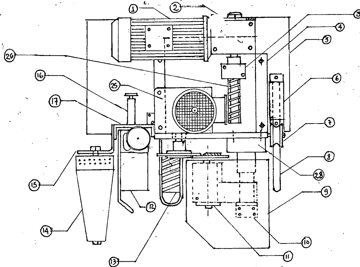
Fig. 1 Vistas Ortogonaes Cortador de Orillo Diseño: Albeiro Gil Fecha : Julio 10/08
