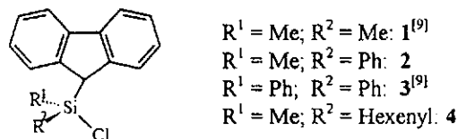
Abb. 1. Dargestellte Fluorenyldialkyl chlorosilane.
