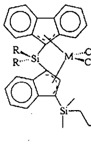
Abb. 5. Übersicht über die dargestellten Metallocendichloridkomplexe.
