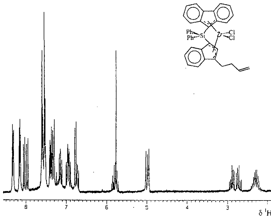
Abb. 6. 250.13 MHz ^1\text{H} -NMR-Spektrum von 36 ( \text{CDCl}_3 , 25°C).
