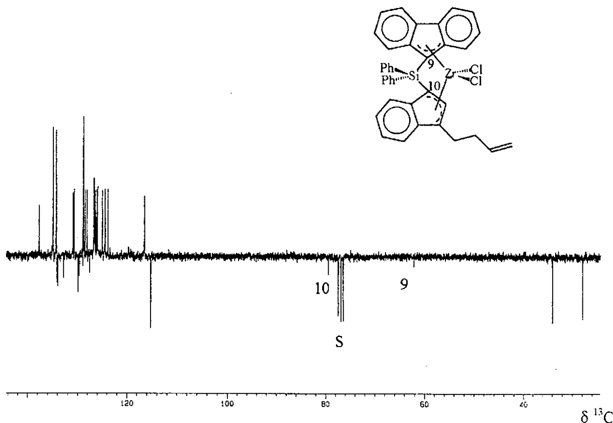
Abb. 7. 62.9 MHz J -moduliertes ^{13}\text{C}\{^1\text{H}\} -NMR-Spektrum von 36 ( \text{CDCl}_3 , 25^\circ\text{C} ). Quartäre und \text{CH}_2 -Kohlenstoffatome (negative Signale) bzw. \text{CH} - und \text{CH}_3 -Kohlenstoffatome (positive Signale) sind in Phase: S = \text{CDCl}_3 .
