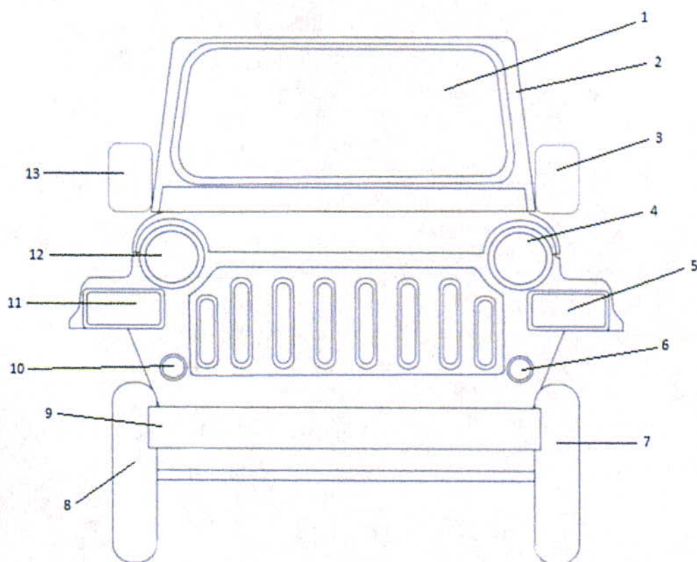
Figura 2. Vista frontal del vehículo eléctrico CE1.
