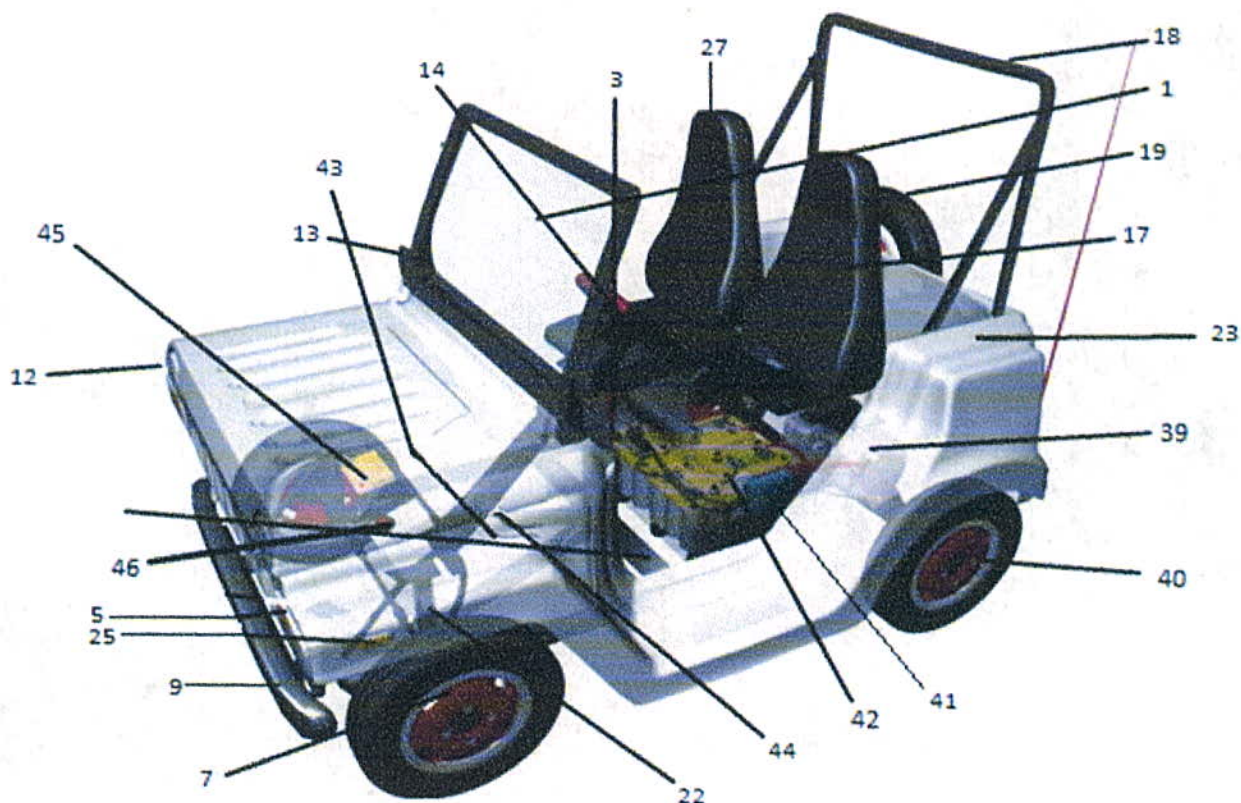
Figura 1. Vehículo CE1
