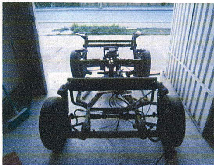
Fotografía 6. Chasis
