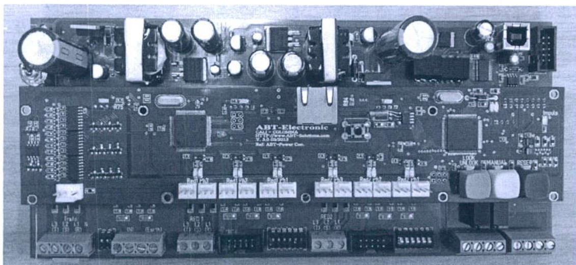
Figura 5. Tarjetas de control y Potencia en Conjunto
