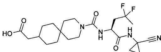
10 ácido {3-[(S)-1-(1-cianociclopropilcarbamoil)-3,3-difluoropentilcarbamoil]-3-azaespiro[5.5]undec-9-il}acético
