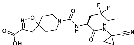
ácido 7-[(S)-1-(1-cianociclopropilcarbamoil)-3,3-difluoro-4-fenilbutilcarbamoil]-1-oxa-2,7-diazaespiro[4.5]dec-2-eno-3-carboxílico
