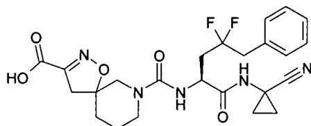
5 ácido 7-[(S)-1-(1-cianociclopropilcarbamoil)-3,3-difluoro-4-fenilbutilcarbamoil]-1-oxa-2,7-diazaespiro[4.4]non-2-eno-3-carboxílico
