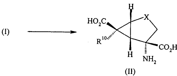
Esquema 1
