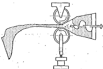
FIGURA 2.34. Esquema de un compactador Chilsonator.
