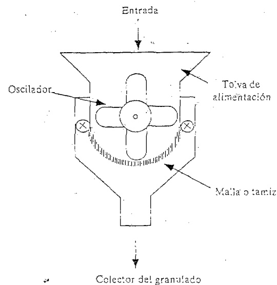
FIGURA 2.28. Esquema de un granulador oscilante.
