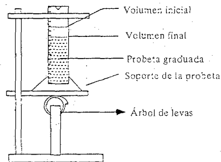
FIGURA. 2.37. Esquema de un voluménometro de asentamiento.
