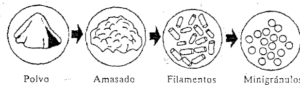
FIGURA 2.32. Diagrama esquemático de un proceso de extrusión/esferonización.
