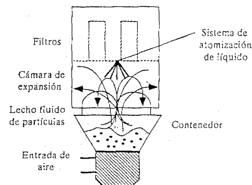
FIGURA 2.29. Granulador de lecho fluido.
