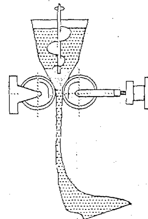
FIGURA 2.34. Esquema de un compactador Chilsonator.
