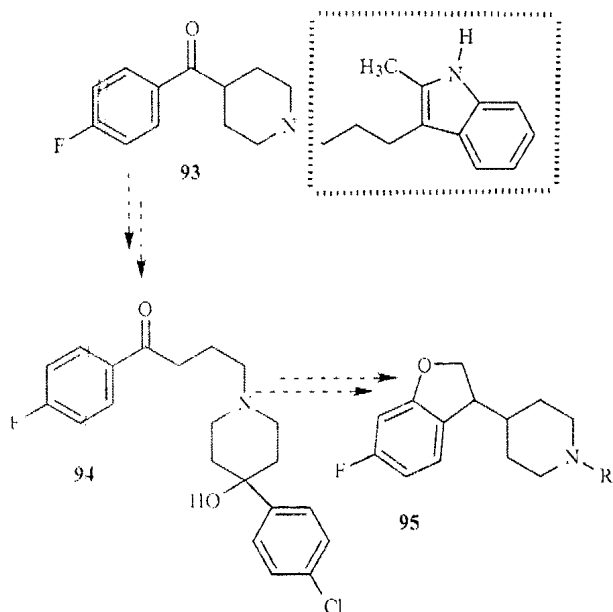
Scheme 26.
