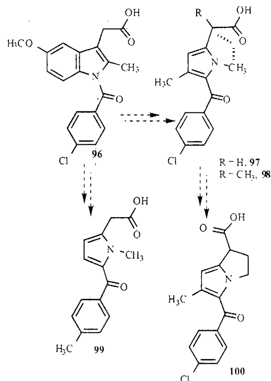
Scheme 27.
