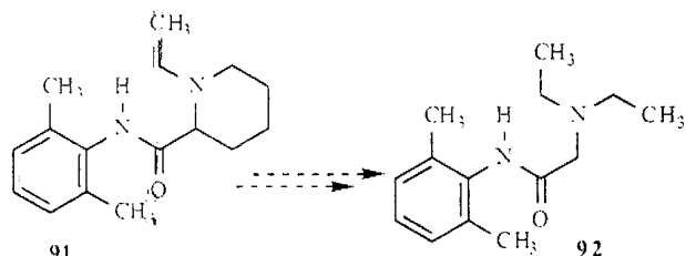
Scheme 25.
