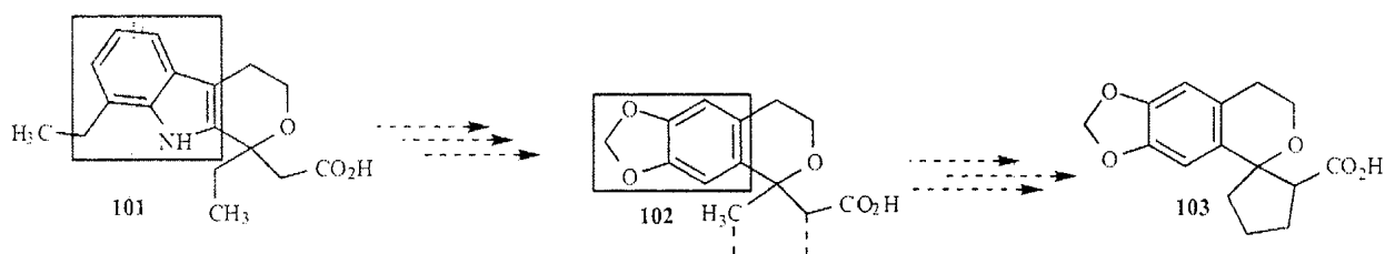
Scheme 28.
