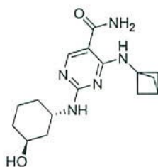
4-(biciclo[1.1.1]pentan-1-ilamino)-2-(((1S,3S)-3-hidroxiciclohexil)amino)pirimidina-5-carboxamida,
