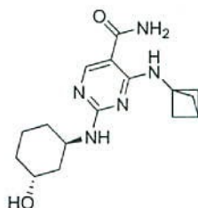
4-(biciclo[1.1.1]pentan-1-ilamino)-2-(((1R,3R)-3-hidroxiciclohexil)amino)pirimidina-5-carboxamida,
