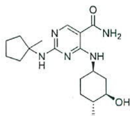
4-(((1R,3R,4R)-3-hidroxi-4-metilciclohexil)amino)-2-((1-metilciclopentil)amino)pirimidina-5-carboxamida,
