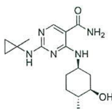
4-(((1R,3R,4R)-3-hidroxi-4-metilciclohexil)amino)-2-((1-metilciclopropil)amino)pirimidina-5-carboxamida,
