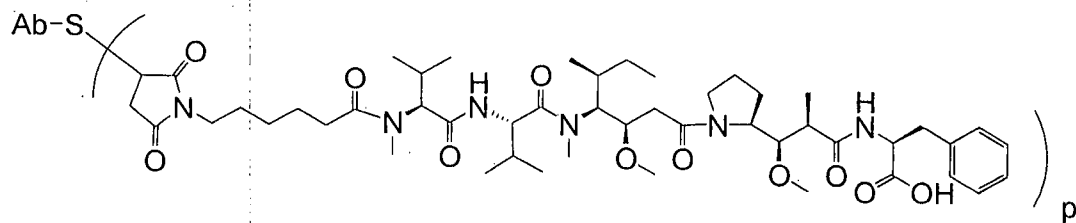
Ab-MC-MMAF
