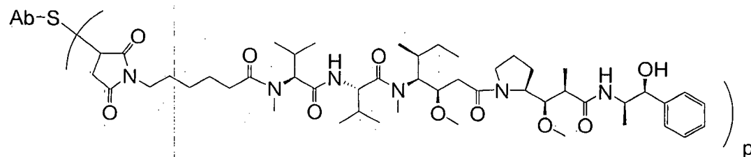
Ab-MC-MMAE
