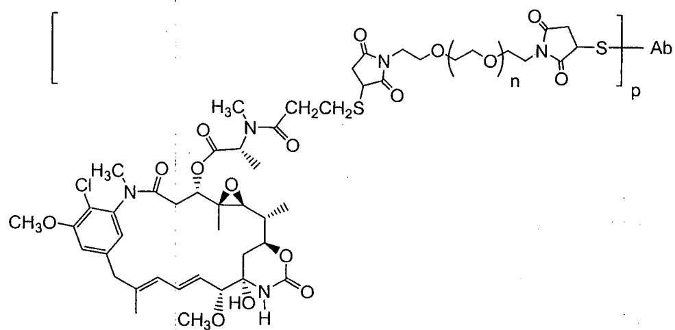
Ab-BMPEO-DM1
