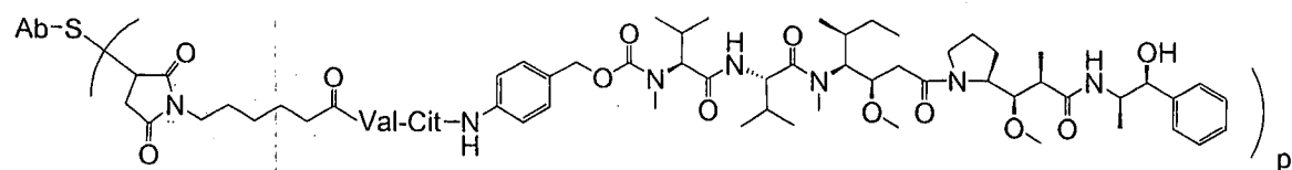
Ab-MC-vc-PAB-MMAE
