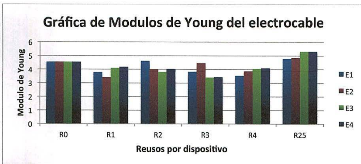
Figura 11. Gráfico de columnas de los cambios en susceptibilidad a la deformación en Mega Pascales (Mpa), para los grupos de lápices de electrocirugía sometidos a 25 reprocesos.
