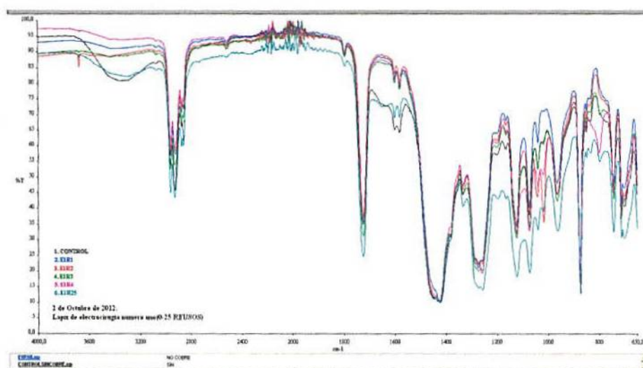
Figura 8. Espectro referencia número uno, espectro de infrarrojos para Policloruro de Vinilo(PVC) con Caucho de Nitrilo(NBR).
