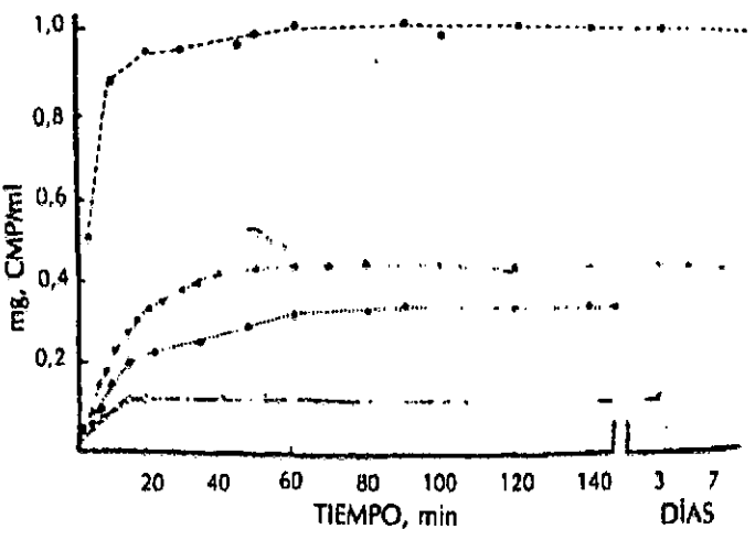
Fig. 76-14. Curvas de disolución de los polimorfos A y B de palmitato de cloranfenicol en alcohol i -butílico al 35% y agua 30 y 38°. Clave: Polimorfo A, 30°, ○—○; polimorfo B, 30°, △—△; polimorfo A, 38°, ●—●; polimorfo B, 38°, ◆—◆.
