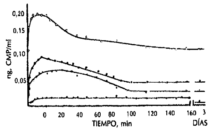
Fig. 76-13. Curvas de disolución del polimorfo C de palmitato de cloranfenicol en alcohol i -butílico al 35% y agua a 30, 20, 15 y 6°. Clave: 30°, ○—○; 20°, ■—■; 15°, △—△; 6°, ●—●.
