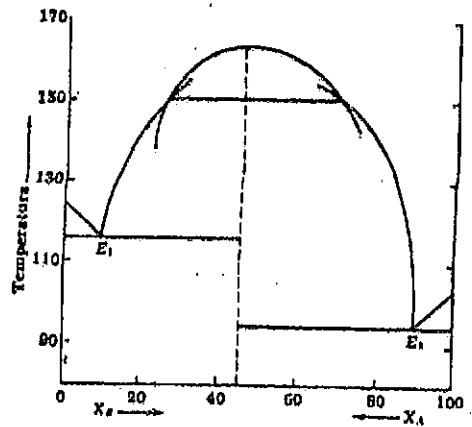
Fig. 30.45. Diagrama de composiciones para 1,3,5-trinitrobenzén (A) y fenantreno (B) mostrando el polimorfismo del compuesto de adición (117).
