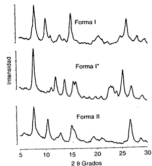
Fig. 83-9. Difractogramas de rayos X para las Formas I, I* y II de SK&amp;F 30097.
