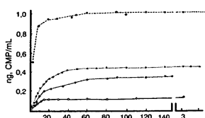
Fig. 83-14. Curvas de disolución de los polimorfos A y B del palmitato de cloramfenicol en alcohol i-butílico al 35% y en agua a 30°C y 38°C. Símbolos: polimorfo A, 30°C, ○; polimorfo B, 30°C, □; polimorfo A, 38°C, ◇; polimorfo B, 38°C, ◇.
