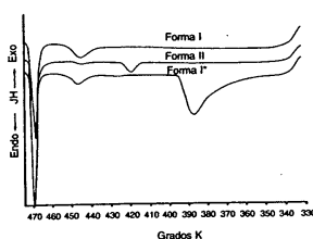
Fig. 83-8. Termogramas para las Formas I, I* e II de SK&F 30097.
