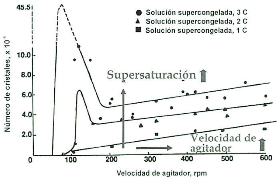
Nucleación Secundaria de Cloruro de Potasio
