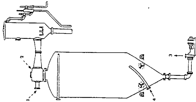
FIG. 30.39. (91). Cristalizador al vacío con reforzador de presión o ejetor de vapor. 1, vapor; 2, refrigerador ejetor; 3, descarga; 4, alimentación.
