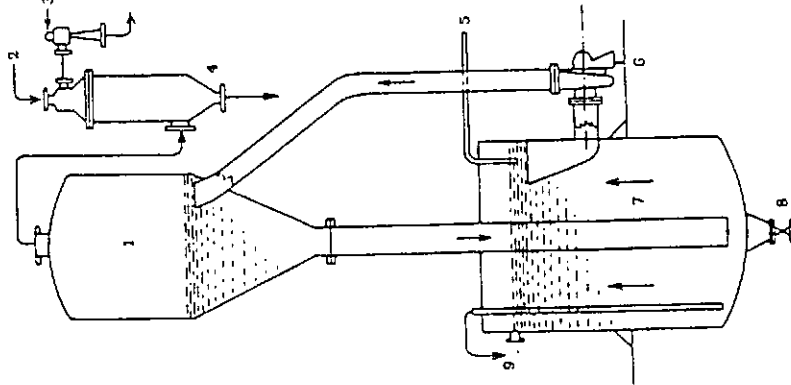
Fig. 30.34. Cristallizador evaporador (91). 1, al condensador; 2, intercambiador de calor; 3, salida del producto; 4, bomba centrífuga; 5, entrada alimentación; 6, cámara de vaporización; 7, suspensión de cristales; 8, difusor; 9, anillo de recirculación.
