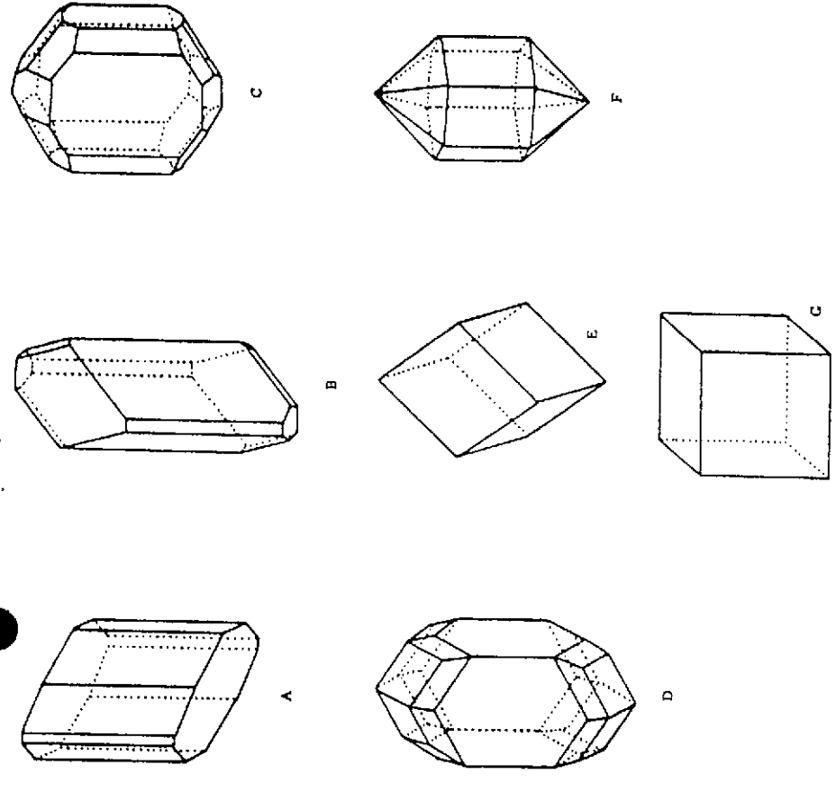
Fig. 30.1. Sistemas cristalográficos. A = triclínico; B = monoclínico; C = ortorrómbico; D = tetragonal; E = romboédrico; F = hexagonal; G = cúbico.
