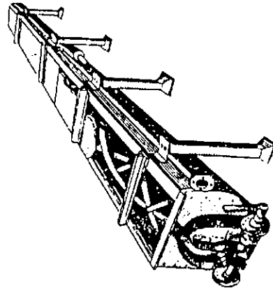
Fig. 30.32. Cristalizador Swenson-Walker.
