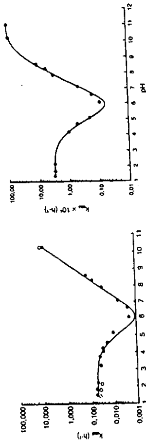
Fig. 83-21. Perfil de la variación de pH para la lactamización de la gabapentina a 80°C y \mu = 0.5M (con NaCl). La línea representa el perfil teórico derivado de la regresión no lineal de cuadrados mínimos de los datos experimentales (●).
