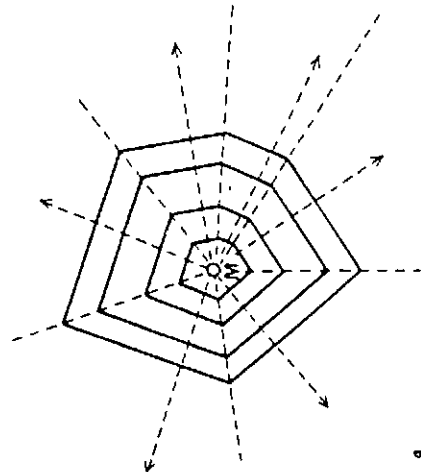
Fig. 30.10. a, crecimiento de las caras de un cristal invariante; b, velocidad de traslación de las caras de un cristal hipotético.
