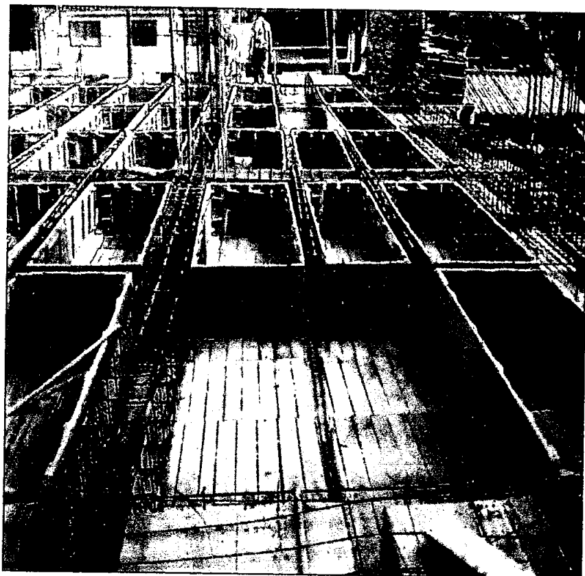
ARMADO DEL CASETON REUTILIZABLE
