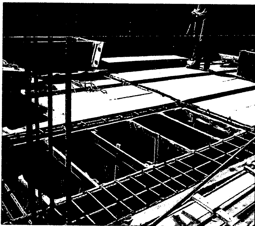
CASETON REUTILIZABLE ARMADO
