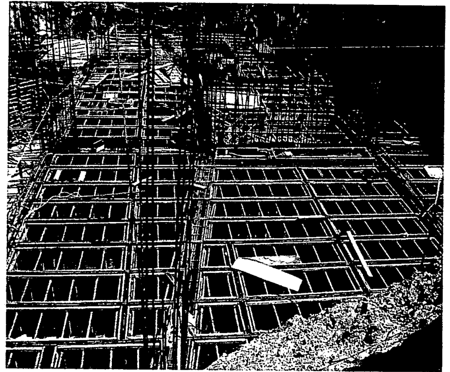
ARMADO DEL CASETON REUTILIZABLE "FRI-HOI"
