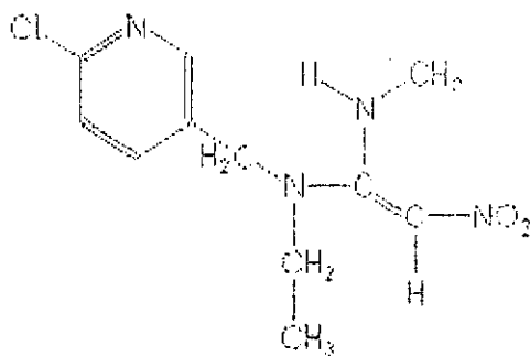
nitenpiram
