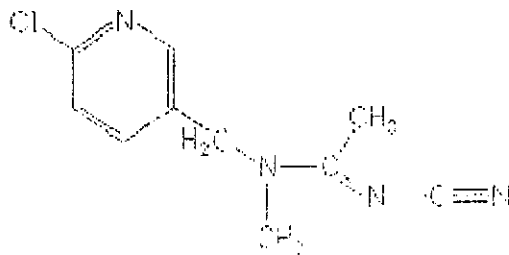
acetamiprid
