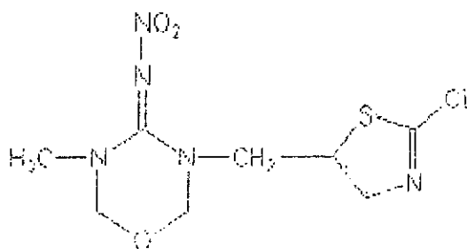
tiameoxan
