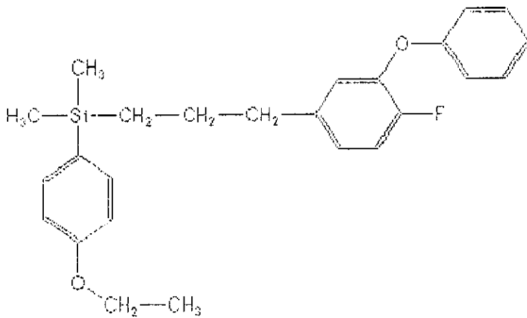
silafuofen
