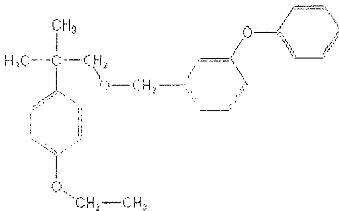
etofenprox
