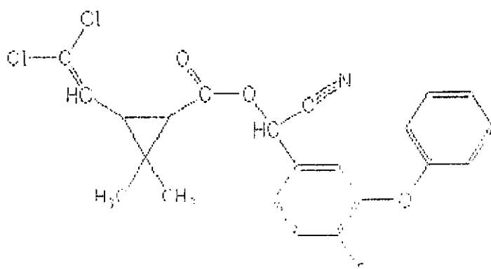
(Z)-(1R)-cis-acid
