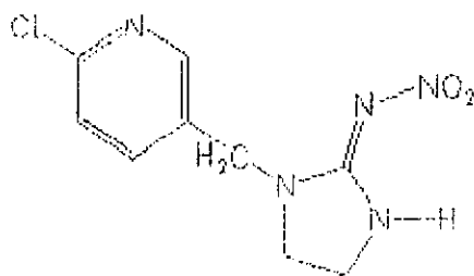
imidacloprid
