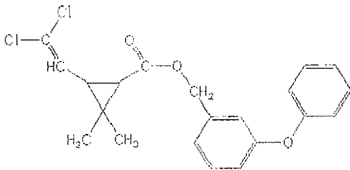
permetrina
