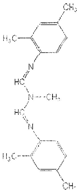
Amitraz
