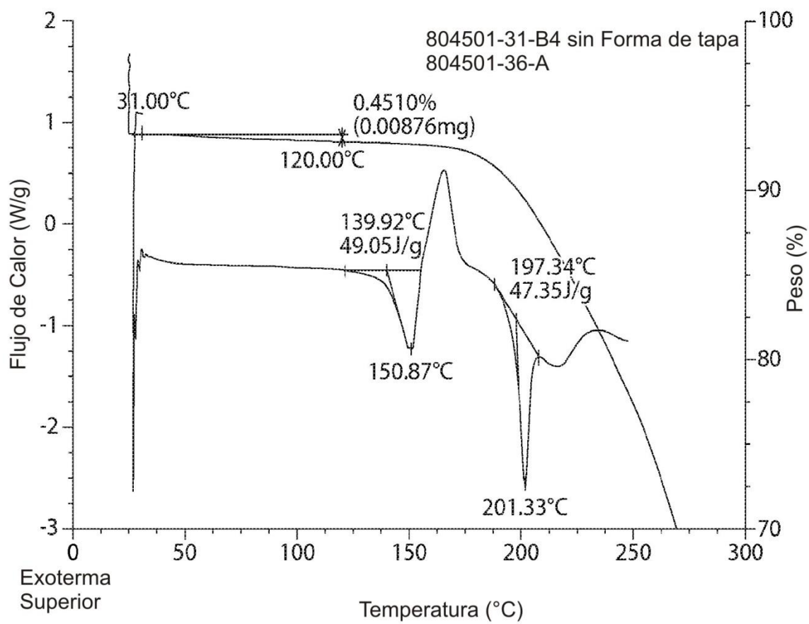
Perfiles de DSC y TGA de la Forma 10
