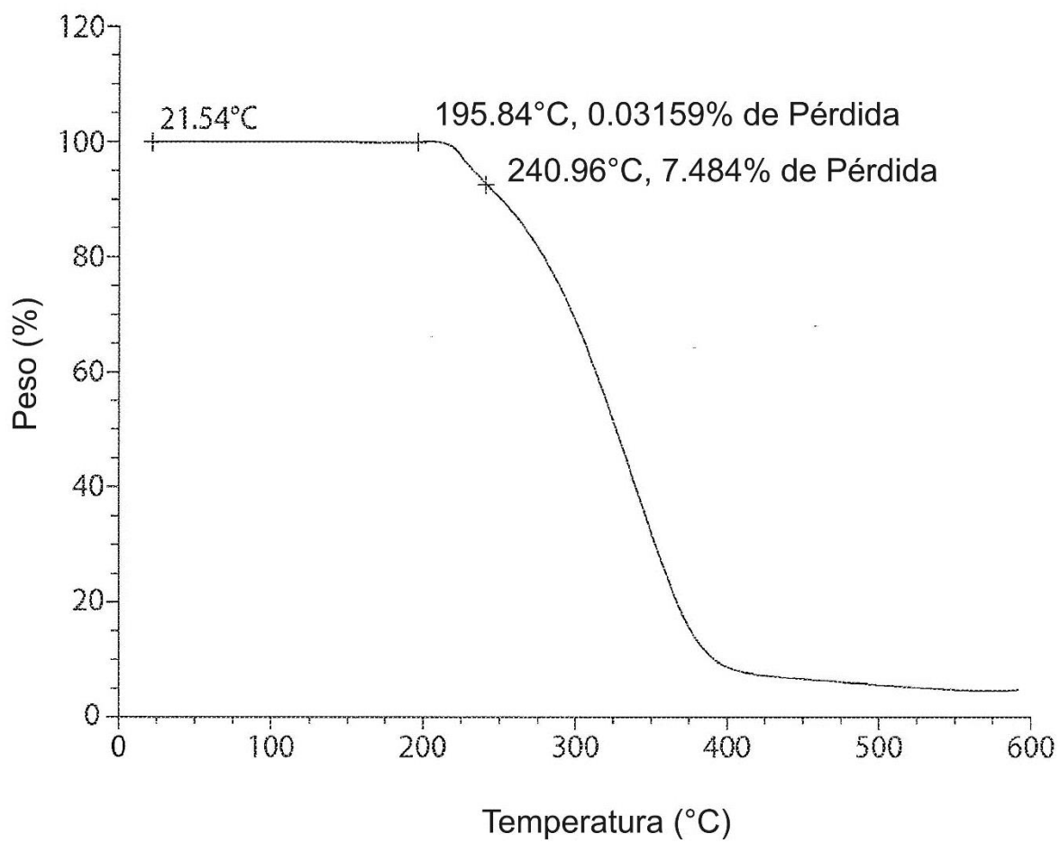
Perfil TGA de la Forma 3
