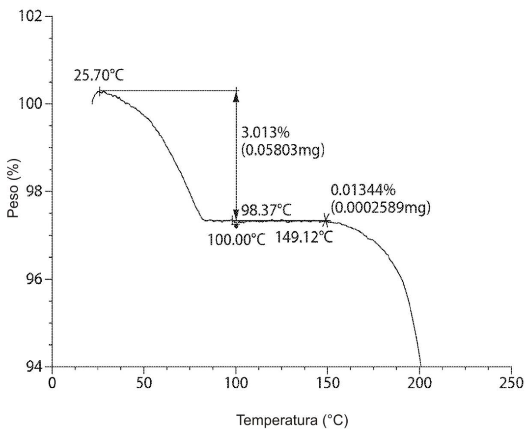
Perfil TGA de la Forma 11
