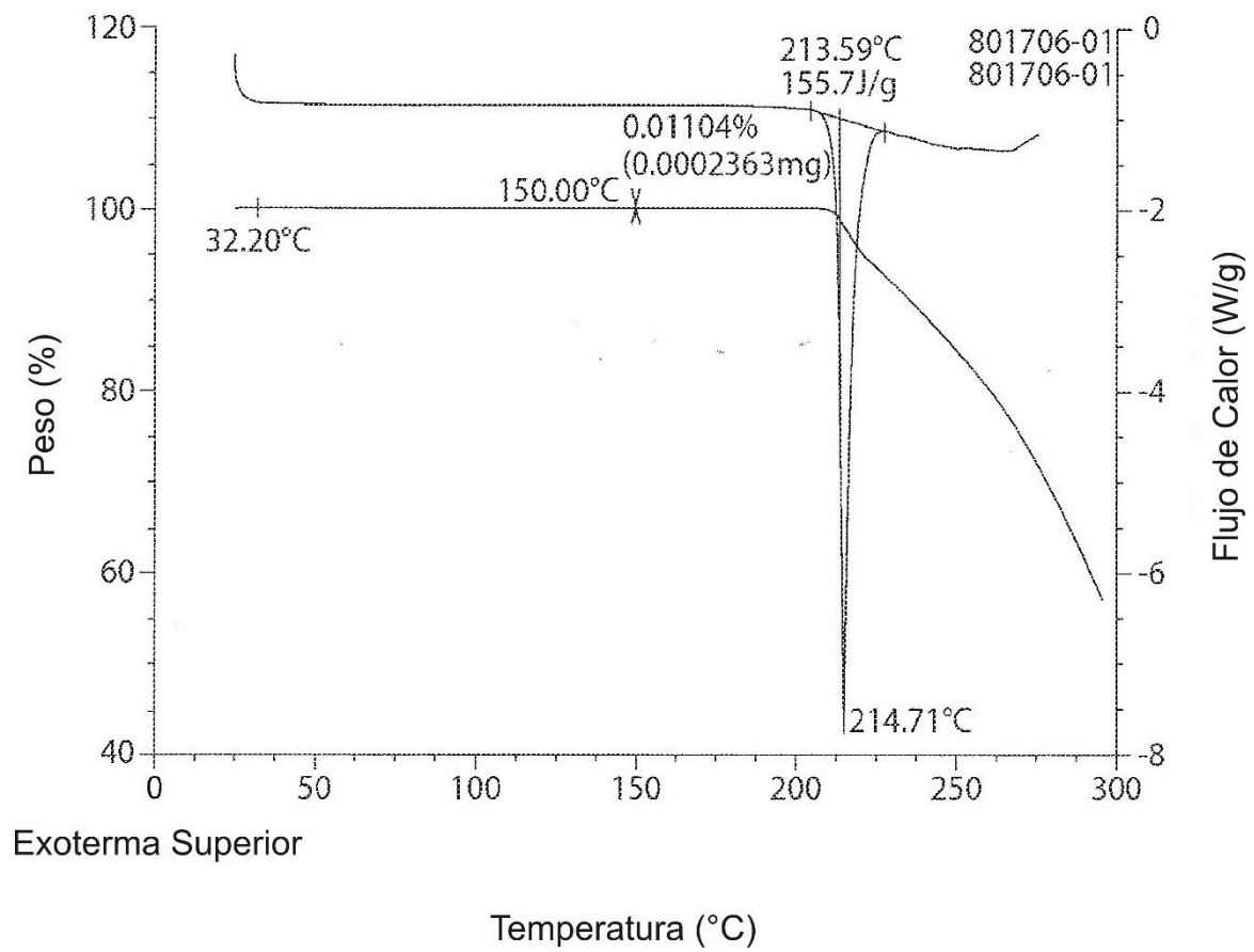
Perfiles de DSC y TGA de la Forma 7
