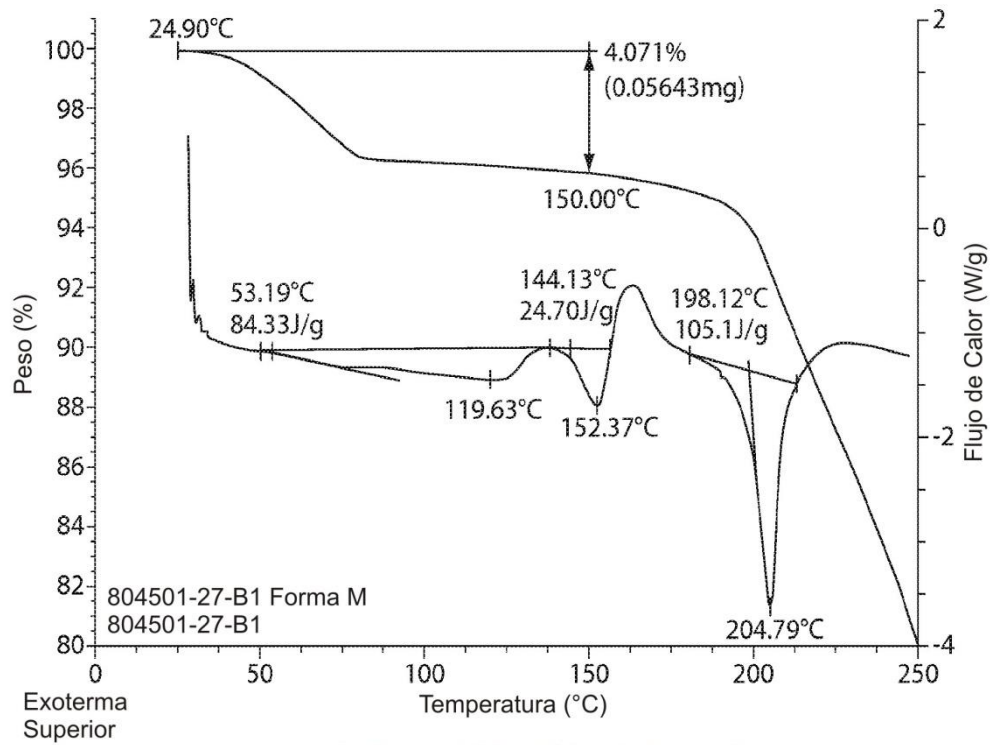
Perfiles de DSC y TGA de la Forma 13
