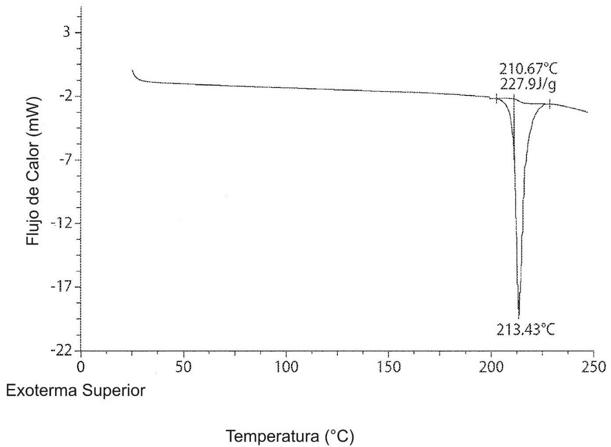
Perfil de DSC de la Forma 3
