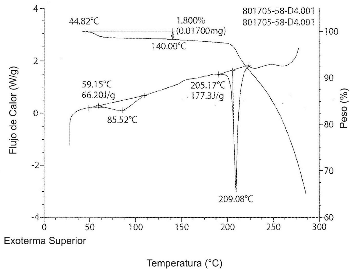
Perfiles de DSC y TGA de la Forma 4
