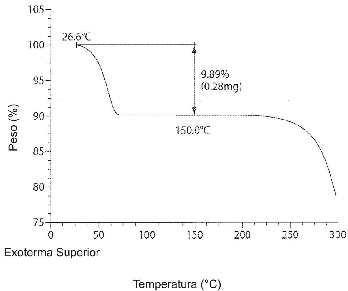
Perfil TGA de la Forma 2
