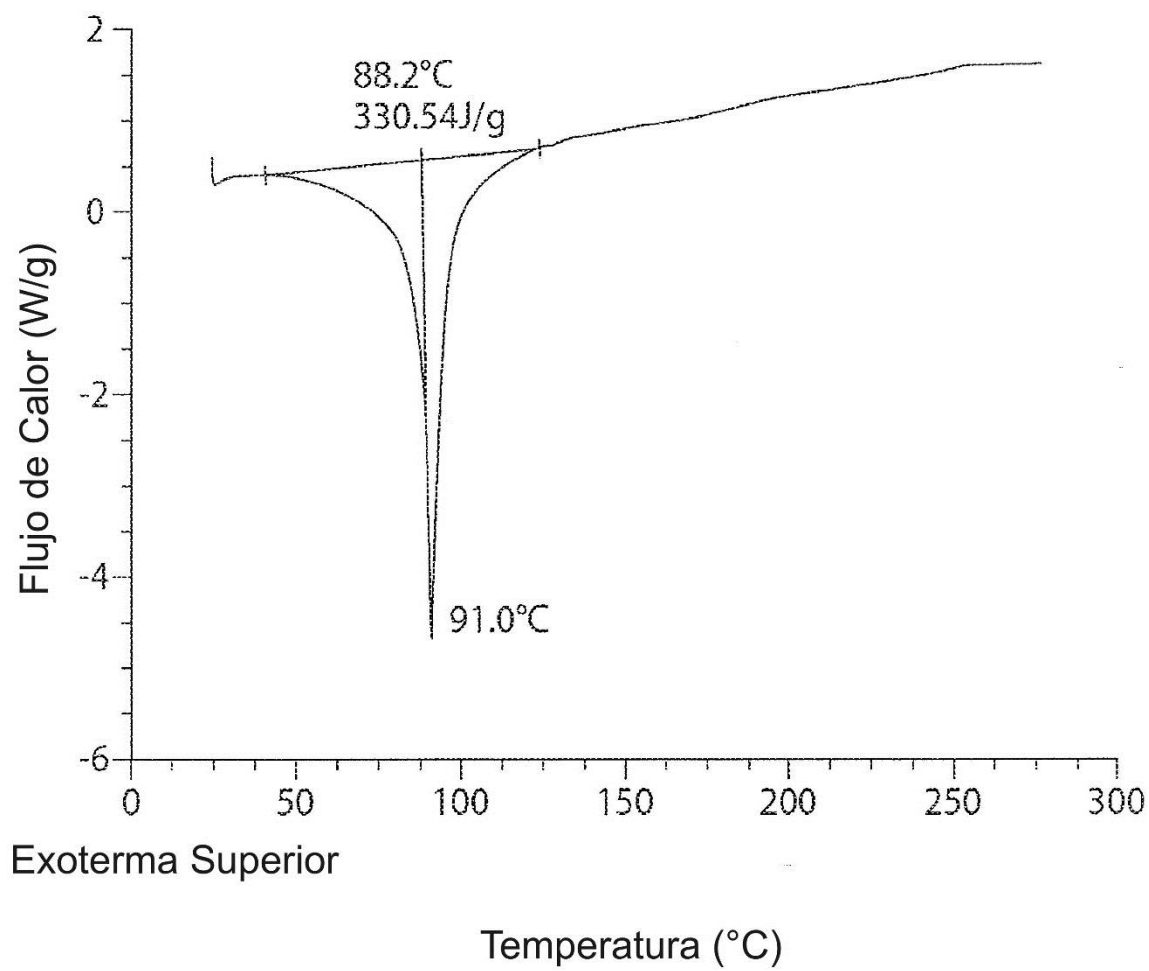
Perfil de DSC de la Forma 2
