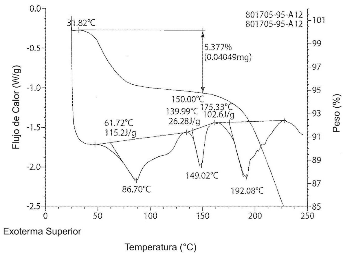
Perfiles de DSC y TGA de la Forma 6
