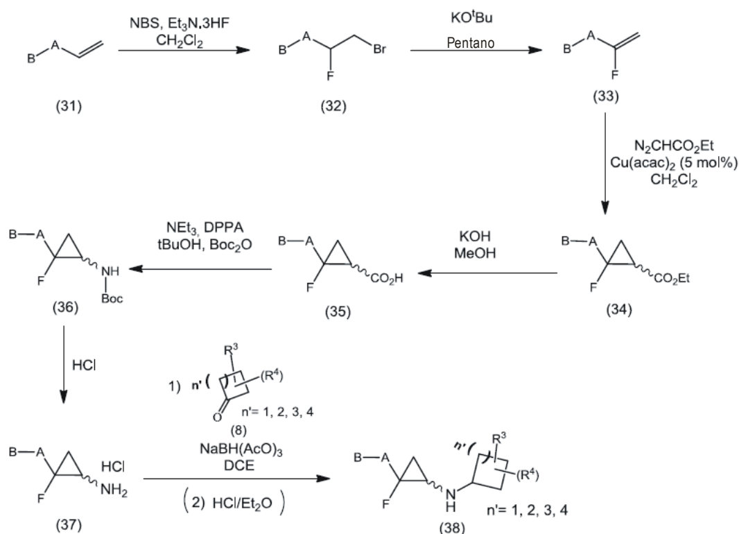
ESQUEMA 6: Boc 2 O (dicarbonato de di-terc-butilo), DCE (dicloroetano), DPPA (difenilfosforil azida), Cu(acac) 2 (acetilacetato de cobre (II) ), NBS (N-bromosuccinimida).
