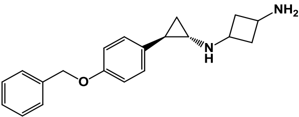
Ejemplo 70: N1-((trans)-2-(3'-(trifluorometil)-[1,1'-bifenil]-4-il)ciclopropil)-2,3-dihidro-1H-indeno-1,3-diamina
