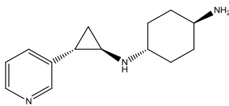
Ejemplo 83: (cis) -N1-((1 R ,2 S )-2-(piridin-3-il)ciclopropil)ciclohexano-1,4-diamina
