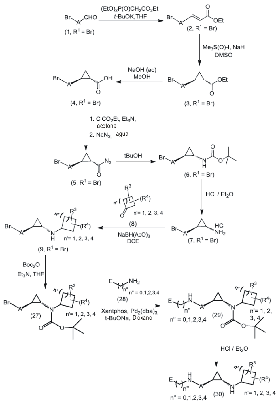
ESQUEMA 5: \text{Boc}_2\text{O} (dicarbonato de di-terc-butilo), DCE (dicloroetano), DMSO (dimetilsulfóxido), \text{Pd}_2(\text{dba})_3 (tris(dibencilidenacetona)dipaladio(0)), THF (tetrahidrofurano), xantfos (4,5-bis(difenilfosfino)-9,9-dimetilxanteno).
