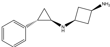
Ejemplo 87: (cis) -N1-((1 R ,2 S )-2-fenilciclo-propil)ciclobutano-1,3-diamina
