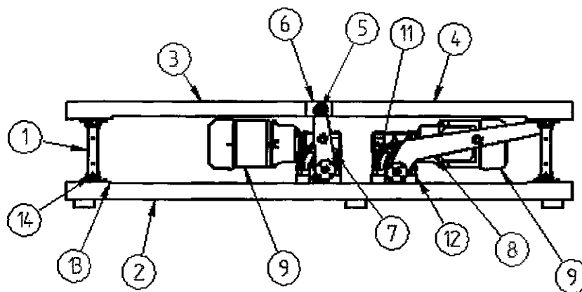
Figura 1. Diseño Mecánico
