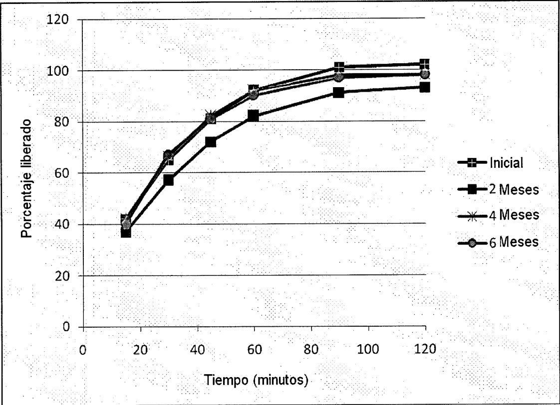
Figura 2. Disolución promedio de masticables de 2 g guardados a 40°C/75% de RH
