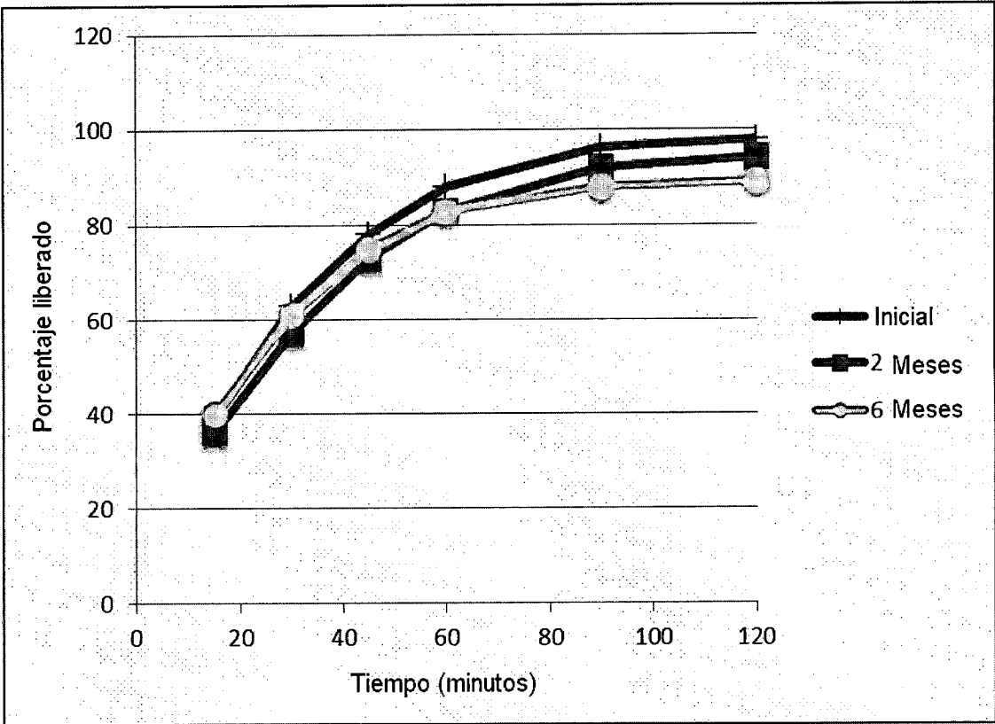
Figura 4. Disolución promedio de masticables de 4 g guardados a 40°C/75% de RH
