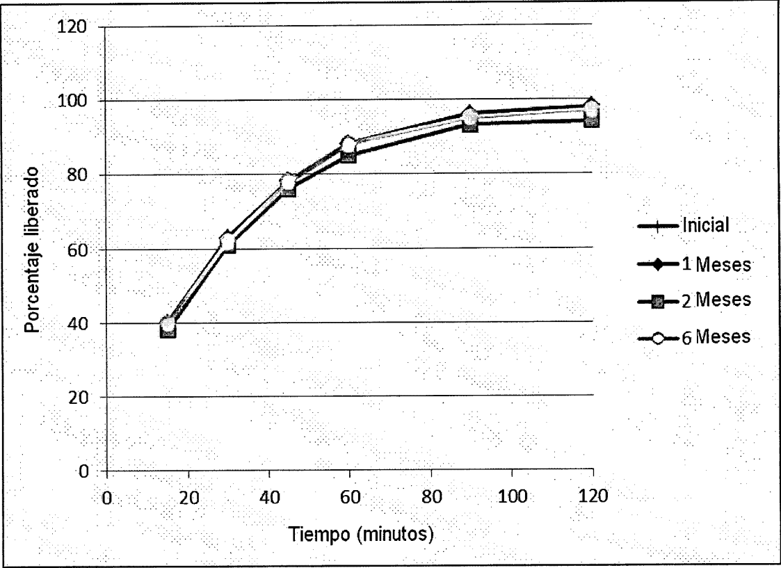
Figura 3. Disolución promedio de masticables de 4 g guardados a 25°C/60% de RH
