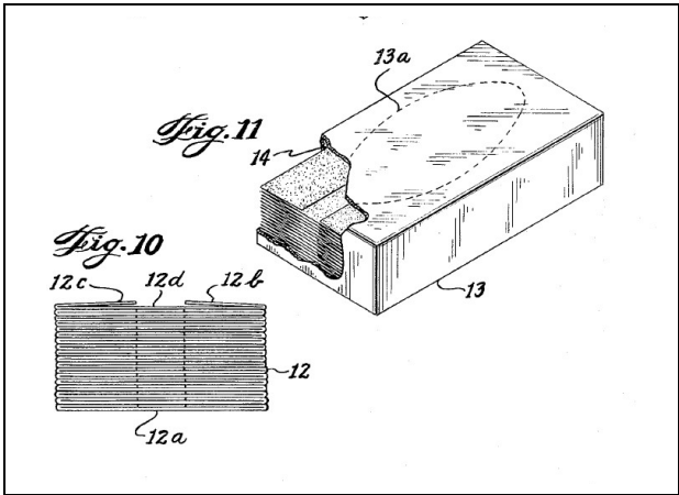
Fig. 10 y 11 D1 (US 3,172,563)
