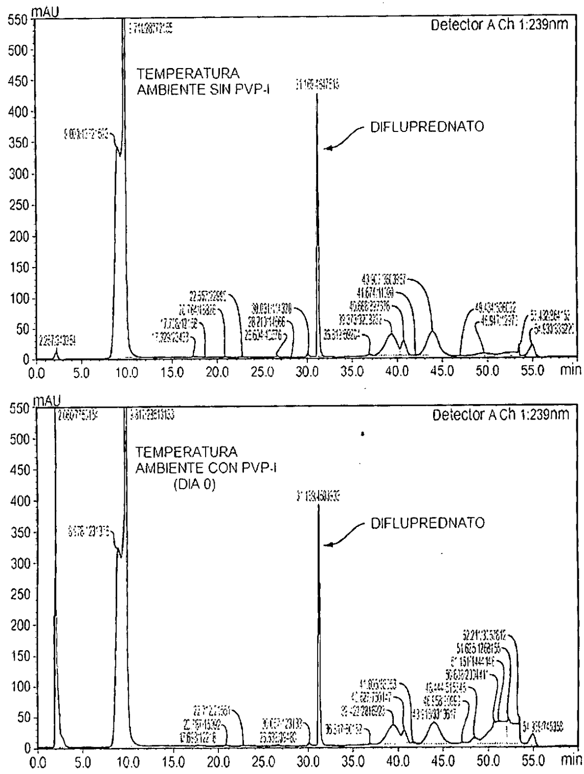
Cromatogramas HPLC-UV del difluprednato en PVP-I para el Día 0
