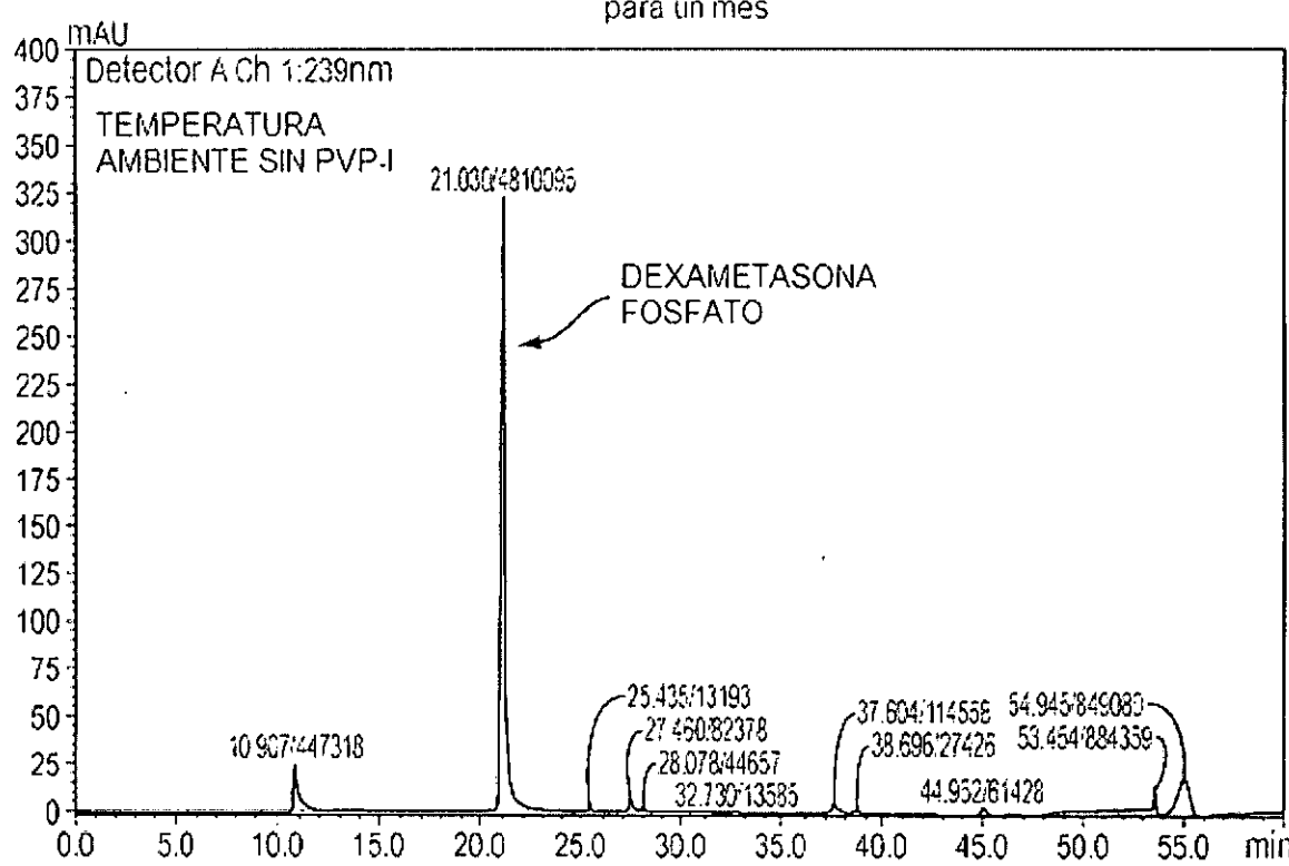
Cromatogramas HPLC-UV del fosfato de dexametasona sodio en PVP-I para un mes
