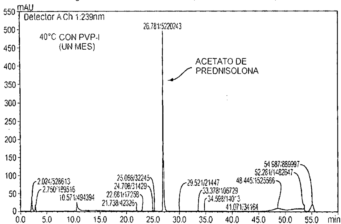
Cromatogramas HPLC-UV del acetato de prednisolona en PVP-I para un mes
