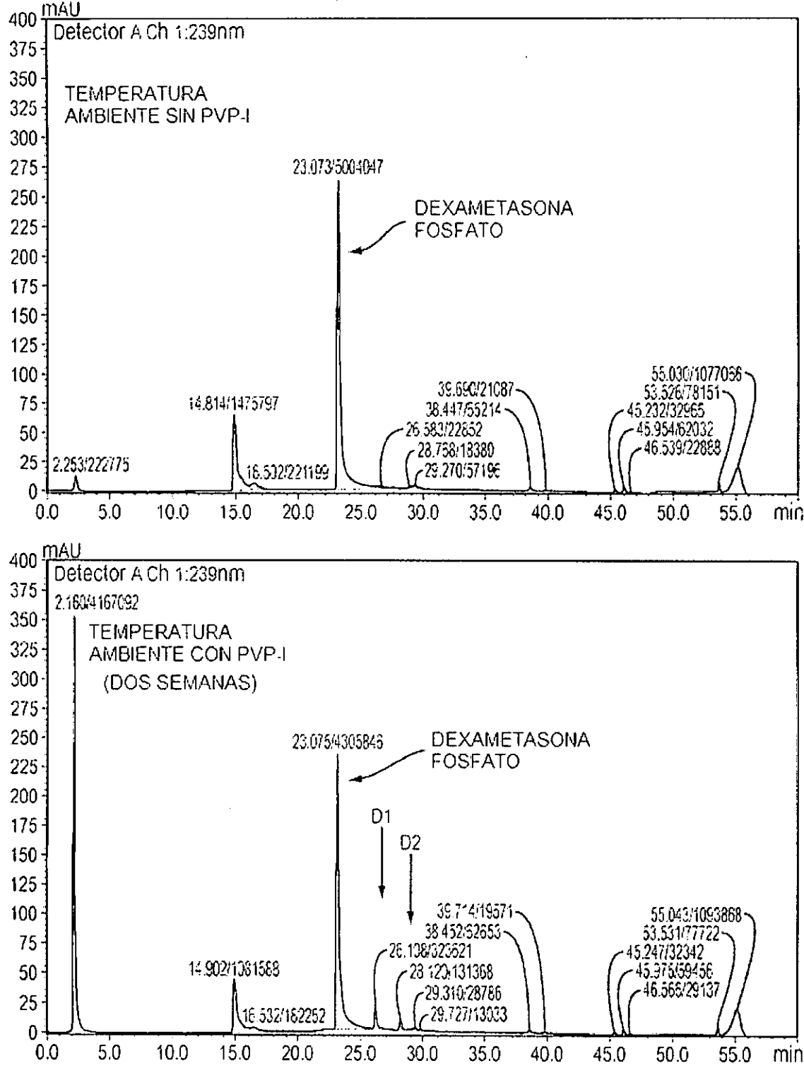
Cromatogramas HPLC-UV del fosfato de dexametasona sodio en PVP-I para dos semanas
