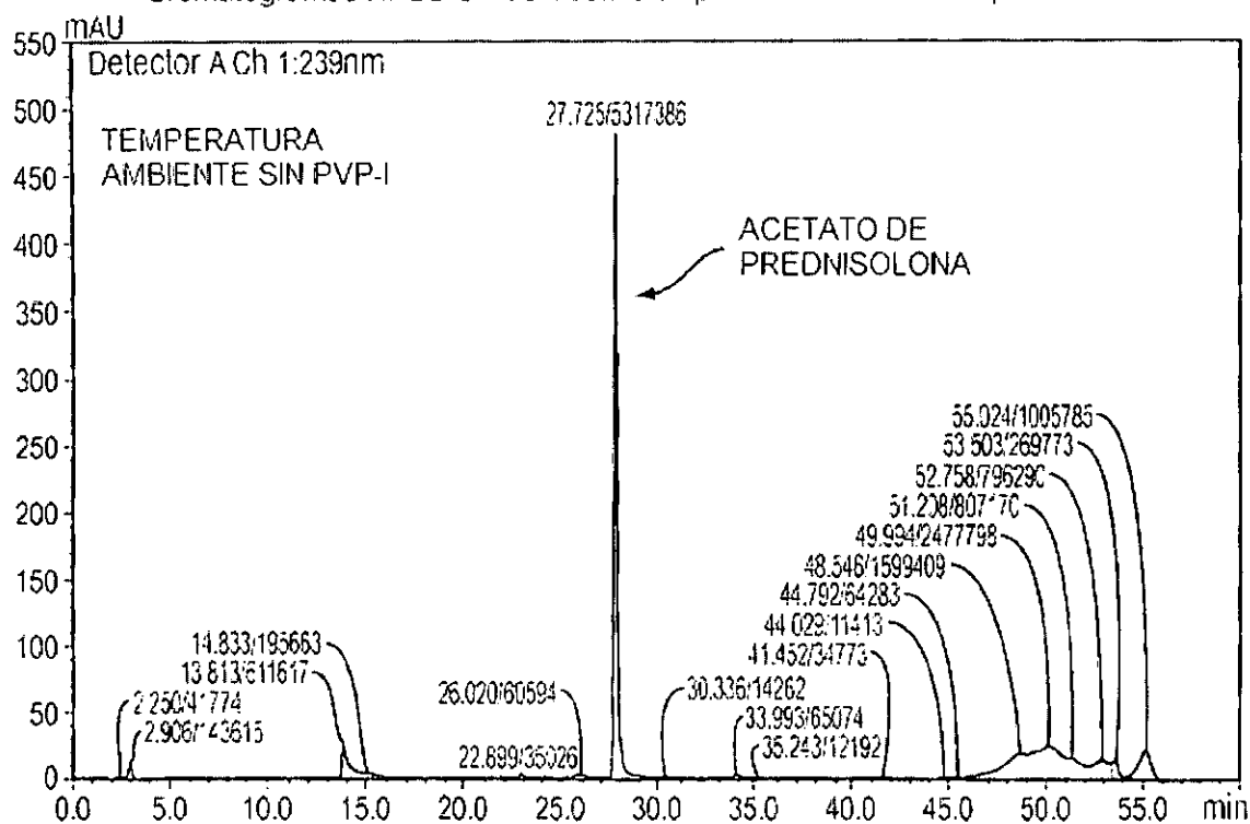
Cromatogramas HPLC-UV del acetato de prednisolona en PVP-I para dos semanas
