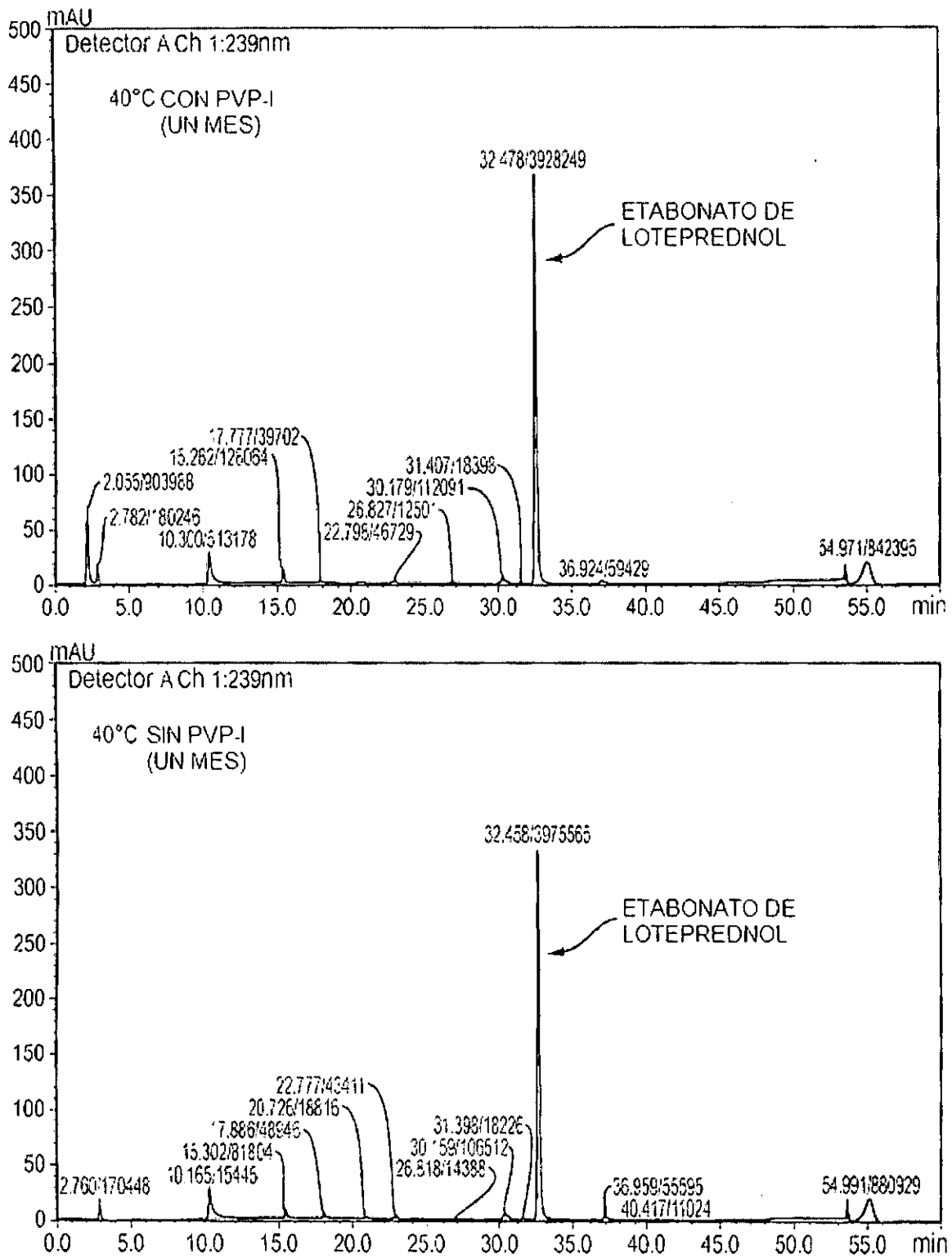
Cromatogramas HPLC-UV del etabonato de loteprednol en PVP-I para un mes
