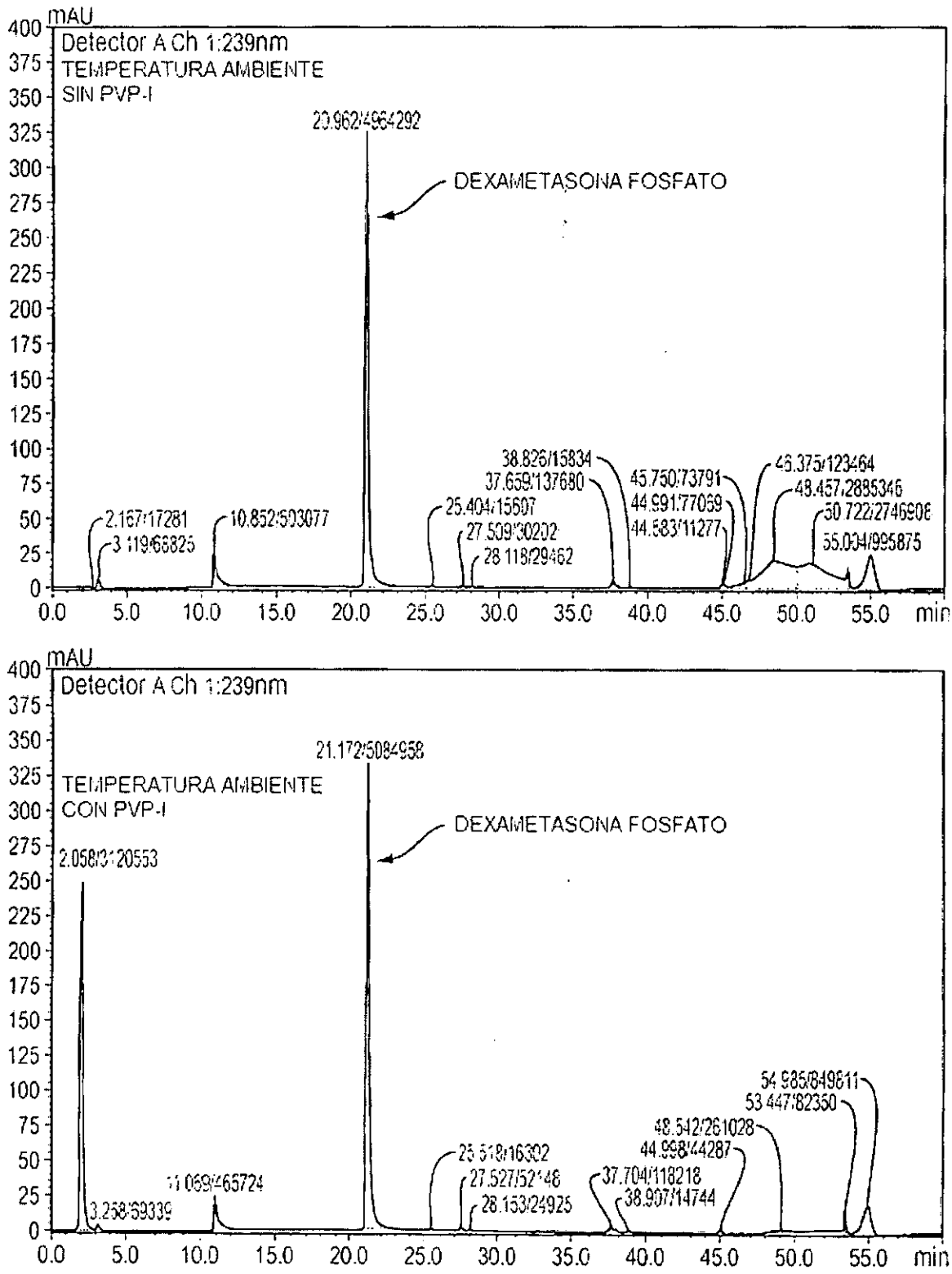
Cromatogramas HPLC-UV del fosfato de dexametasona sodio en PVP-I para el Día 0
