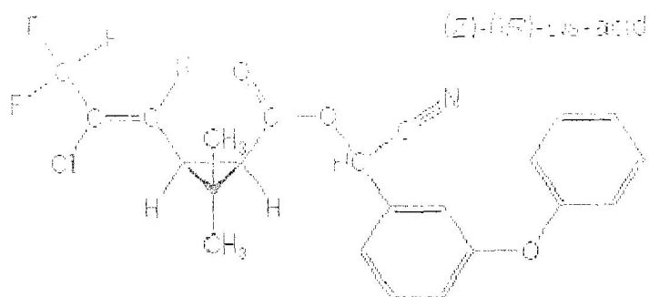
(Z)-(1S)-cis-acid
