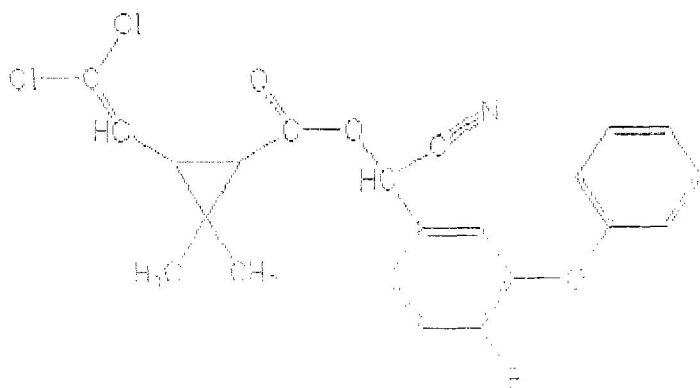
(Z)-(1S)-cis-acid
