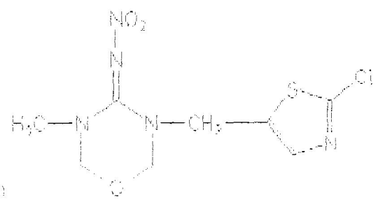
tiametoxan
