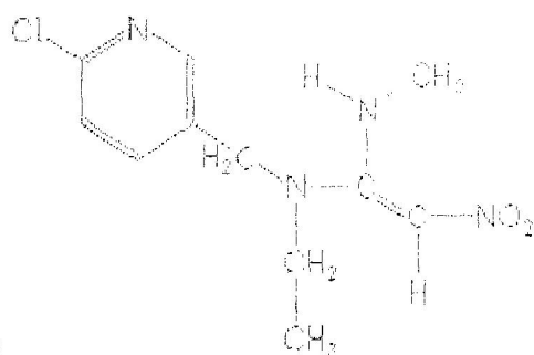
nitompram
