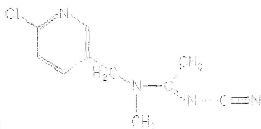
acetamiprid
