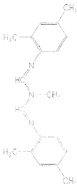
Amitraz
