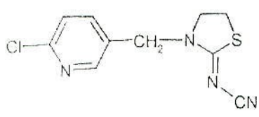
Thiacloprid
