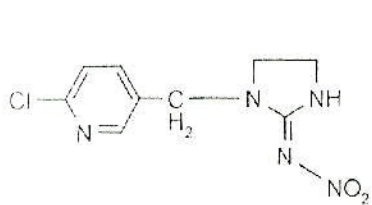
Imidacloprid
