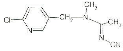
Acetamiprid
