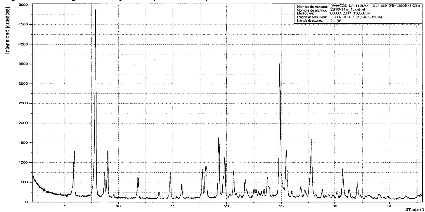
Figura 14: difractogramas de rayos X en polvo del compuesto de la fórmula I como el dihidrato
