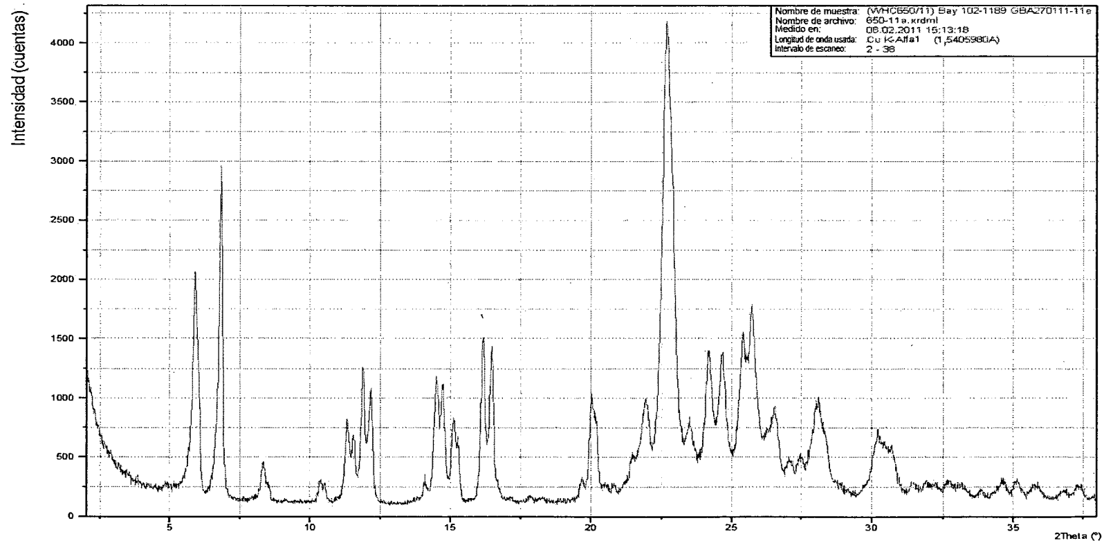
Figura 5: difractogramas de rayos X en polvo del compuesto de la fórmula I en polimorfo I
