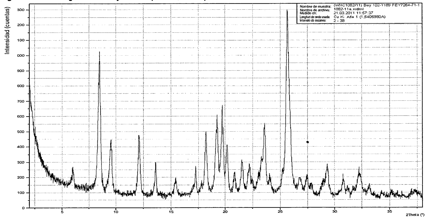
Figura 13: difractogramas de rayos X en polvo del compuesto de la fórmula I como el monohidrato
