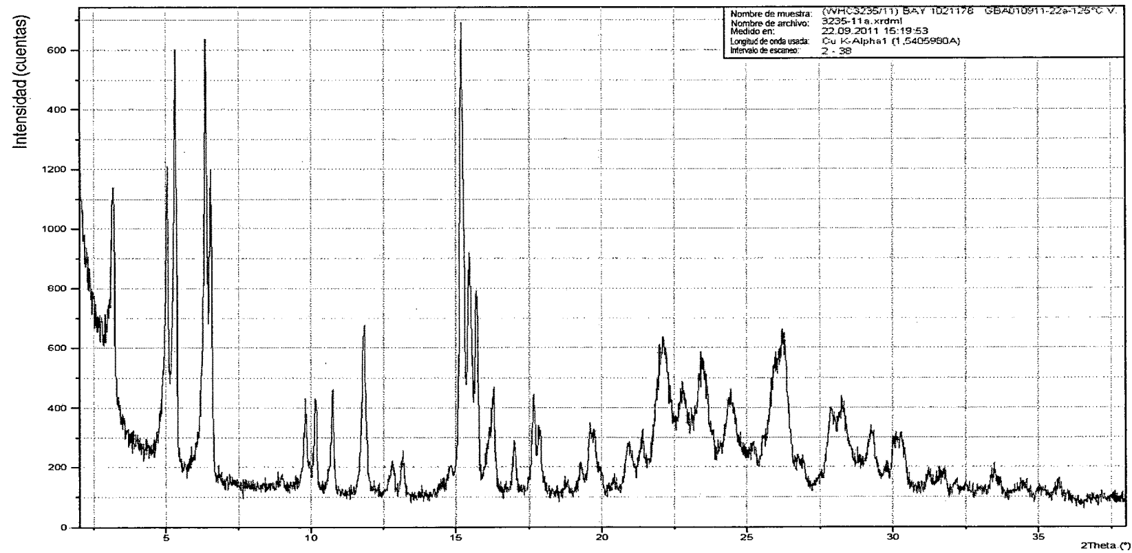
Figura 9: difractogramas de rayos X en polvo del compuesto de la fórmula I en polimorfo V
