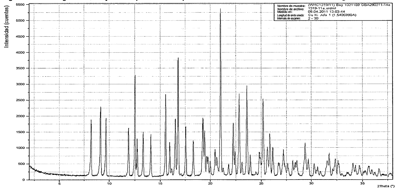
Figura 12: difractogramas de rayos X en polvo del compuesto de la fórmula I como el solvato de DMF-agua
