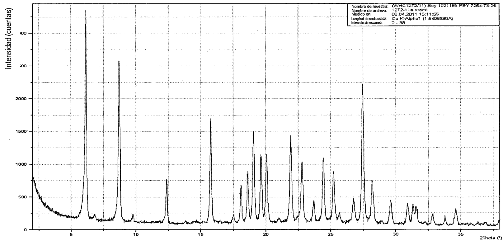
Figura 7: difractogramas de rayos X en polvo del compuesto de la fórmula I en polimorfo III
