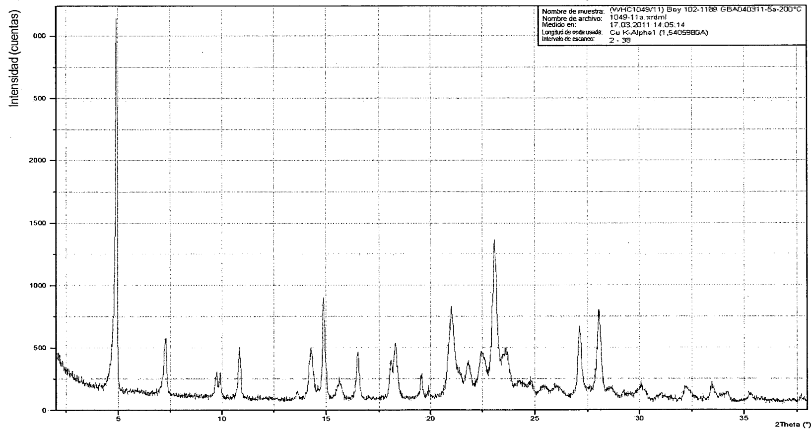
Figura 6: difractogramas de rayos X en polvo del compuesto de la fórmula I en polimorfo II
