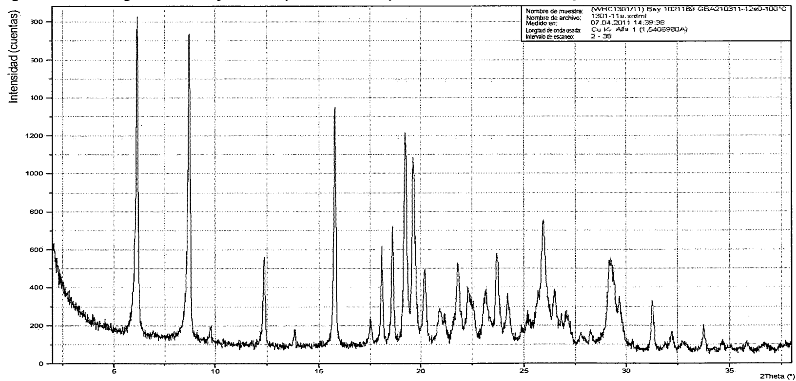
Figura 8: difractogramas de rayos X en polvo del compuesto de la fórmula I en polimorfo IV
