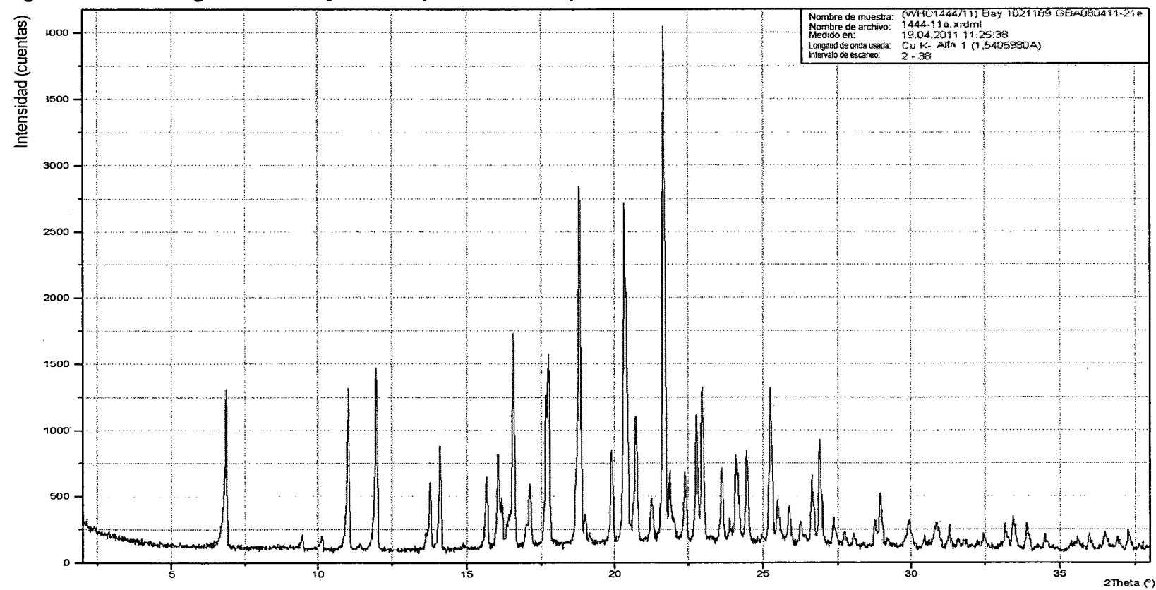
Figura 11: difractogramas de rayos X en polvo del compuesto de la fórmula I como el solvato de di-DMSO
