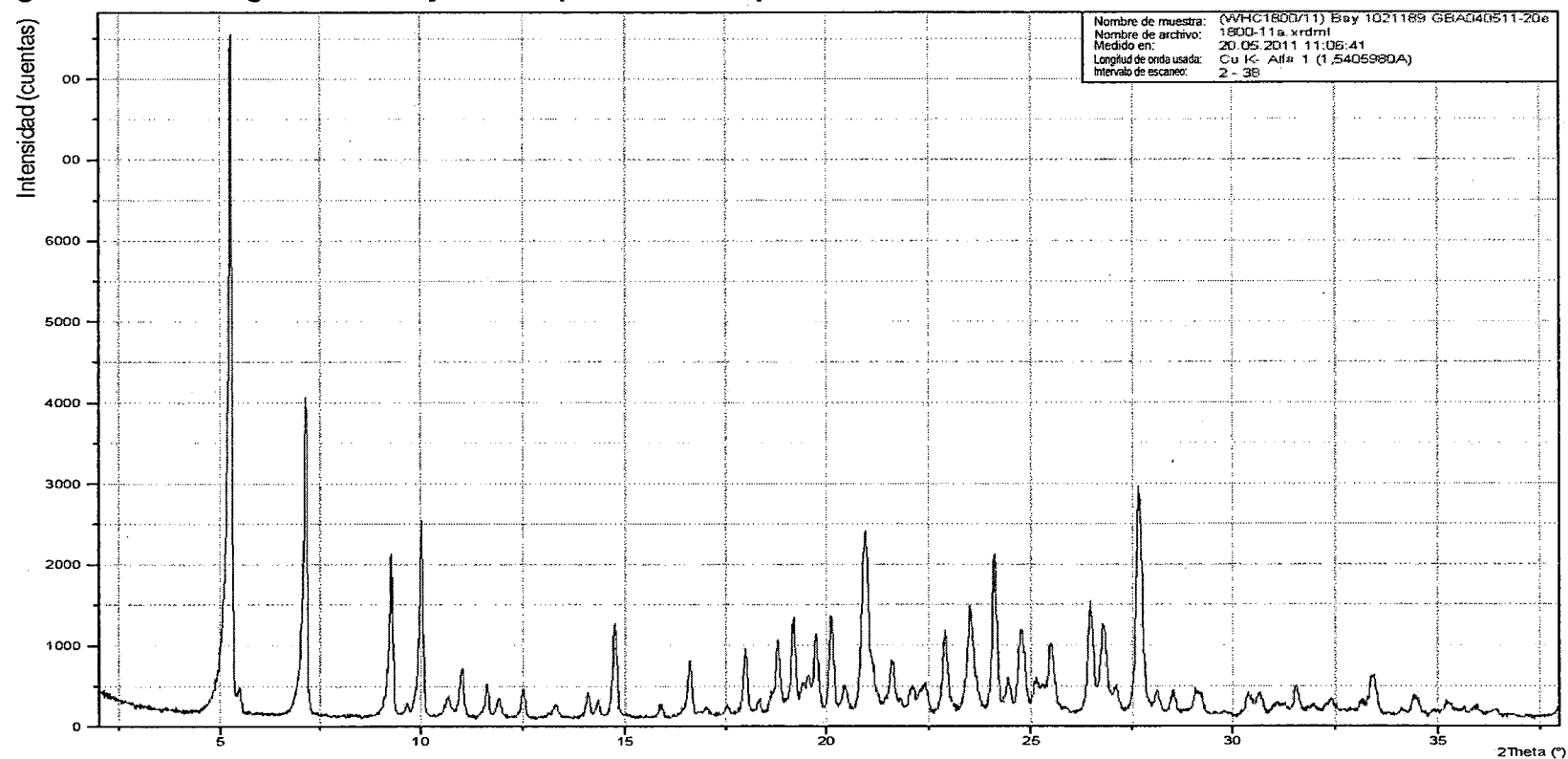
Figura 10: difractogramas de rayos X en polvo del compuesto de la fórmula I como el solvato de ácido triacético
