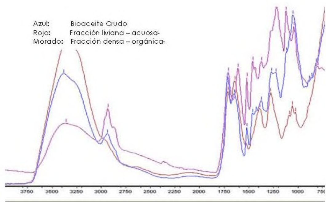
5 Figura 4. Espectro IR bioaceite crudo y productos de hidrotratamiento
