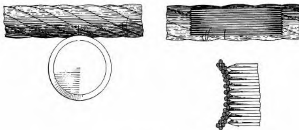
FIGURA 9 (Estado de la técnica)
