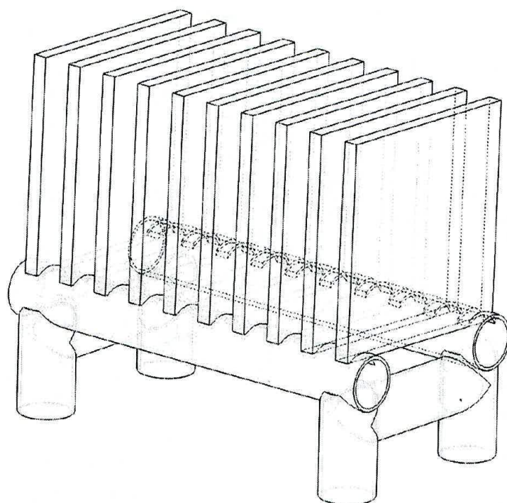
Ensamblado Dispositivo
