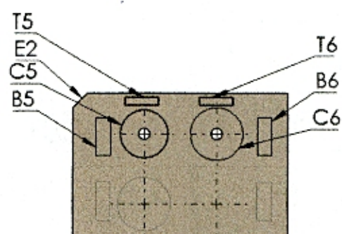
VISTA POSTERIOR
