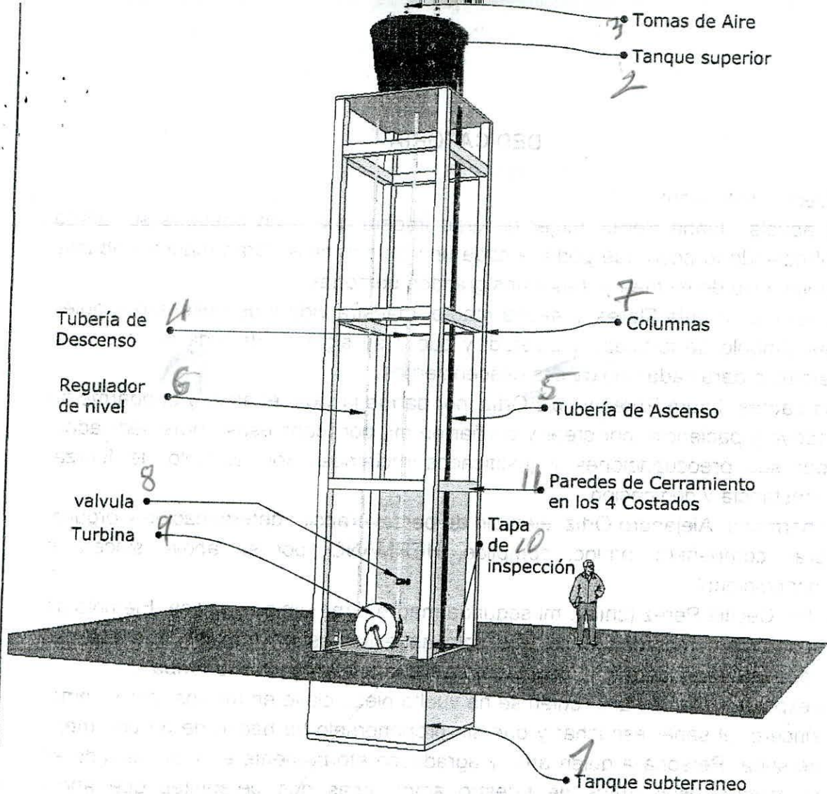
Detalle Sistema
