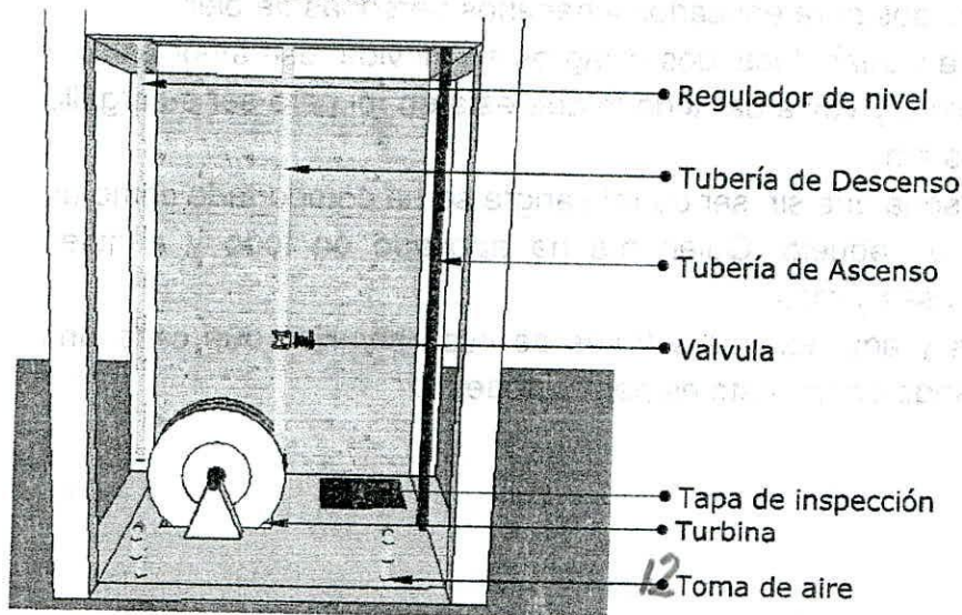
Detalle Sistema
