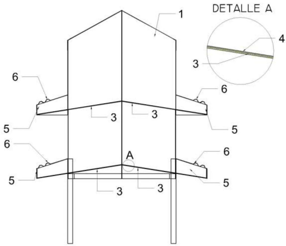
CORTE A-A
