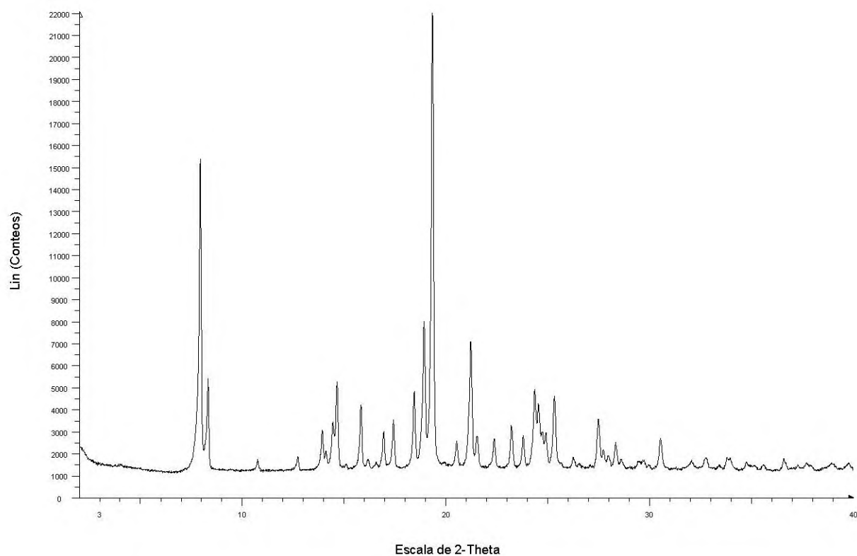
Figura 1: Patrón de difracción de rayos X de polvo de la forma D de (2 S )-2-Metoxi-2- 5 fenil- N -[5-[[[(3 R )-1-piridazin-3-ilpirrolidin-3-il]amino]-1,3,4-tiadiazol-2-il]acetamida.
