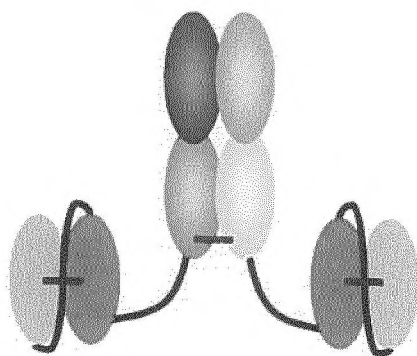
Fab#2-(HC)dsscFv#3-(LC)dsscFv#3
