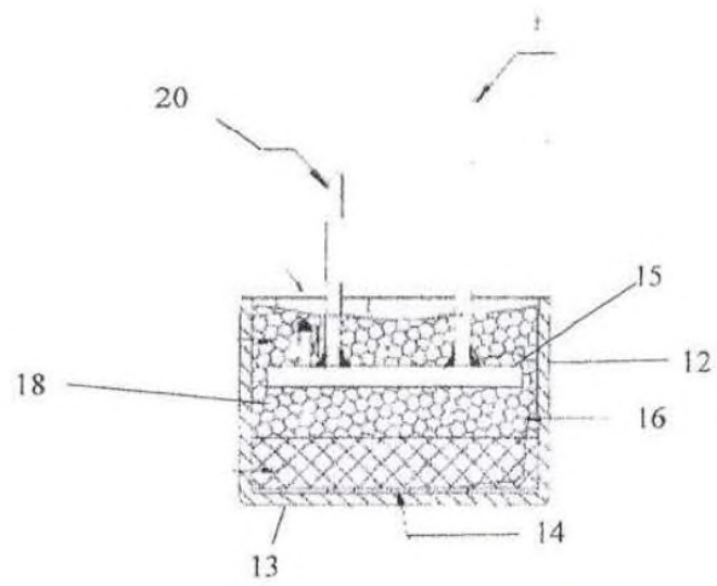
Figura 1. Elemento piezoeléctrico
