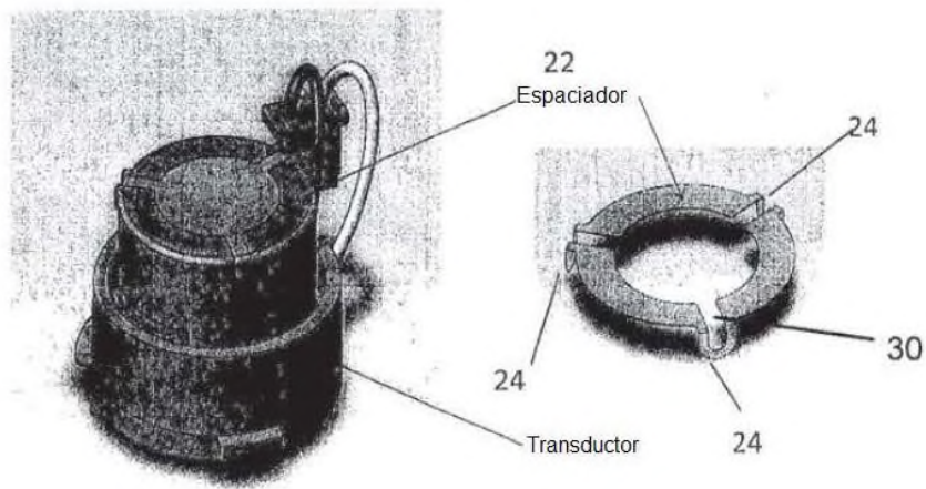
Figura 2: Elemento piezoeléctrico con espaciador
